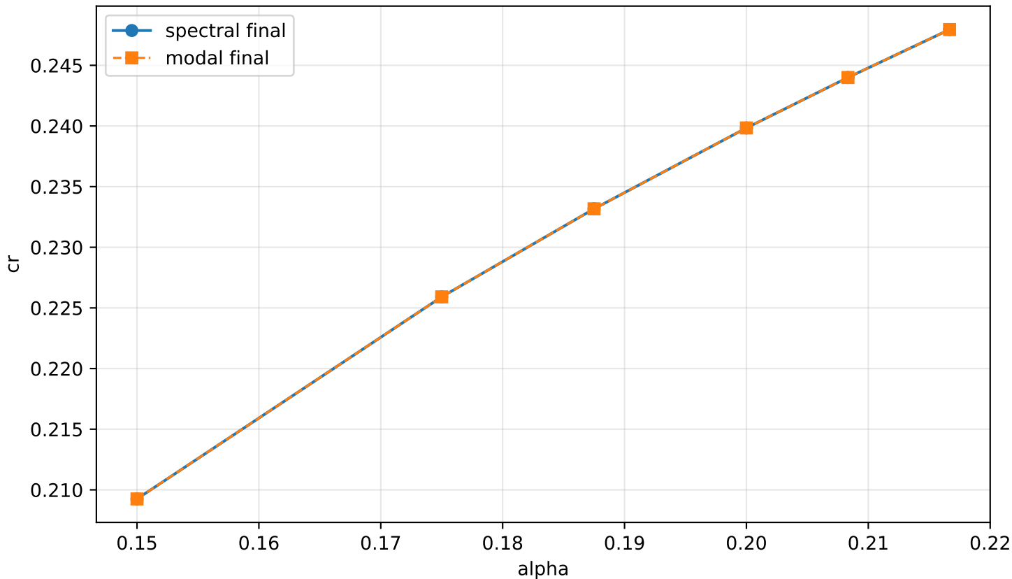
Final23 cr(alpha), M=1.2
