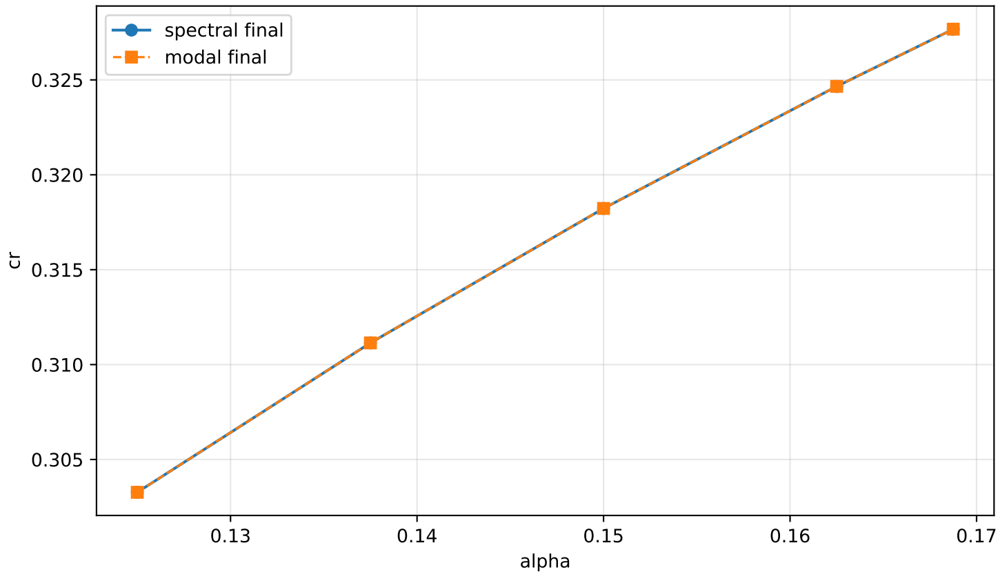
Final23 cr(alpha), M=1.4
