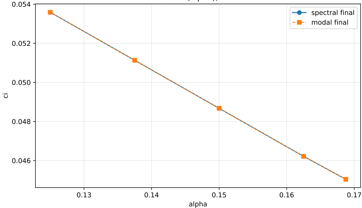
Final23 ci(alpha), M=1.4
