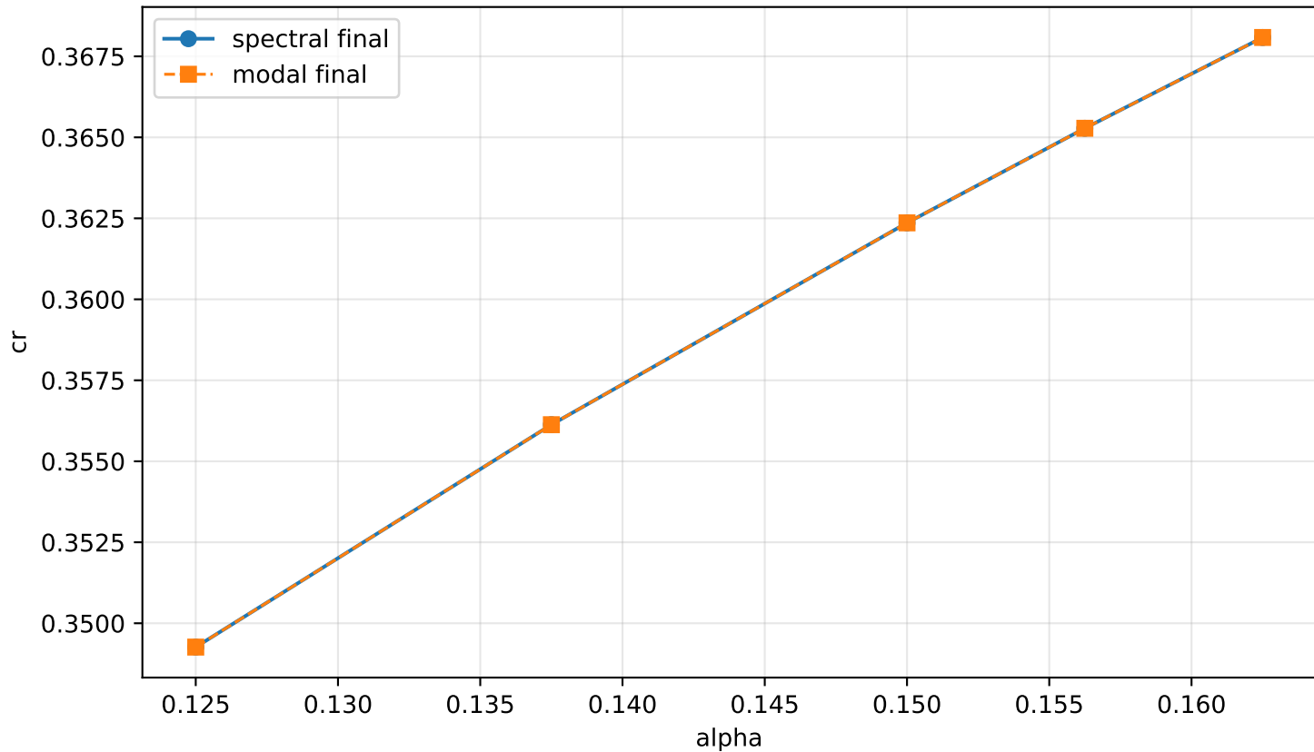
Final23 cr(alpha), M=1.5
