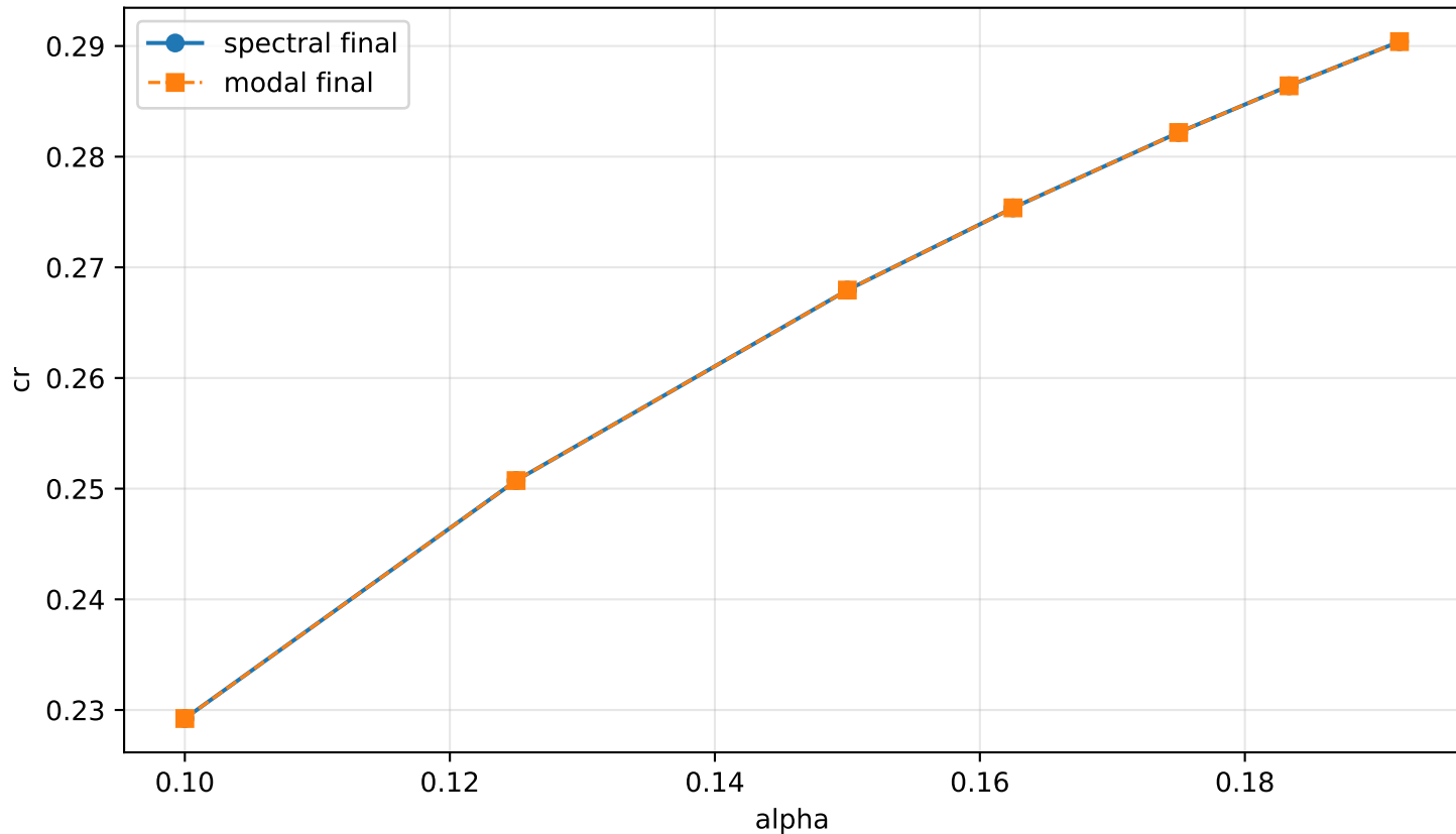
Final23 cr(alpha), M=1.3
