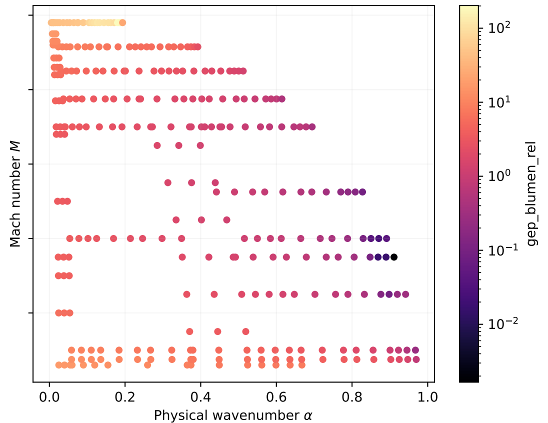
(d) GEP final vs Blumen: stabilized relative error
