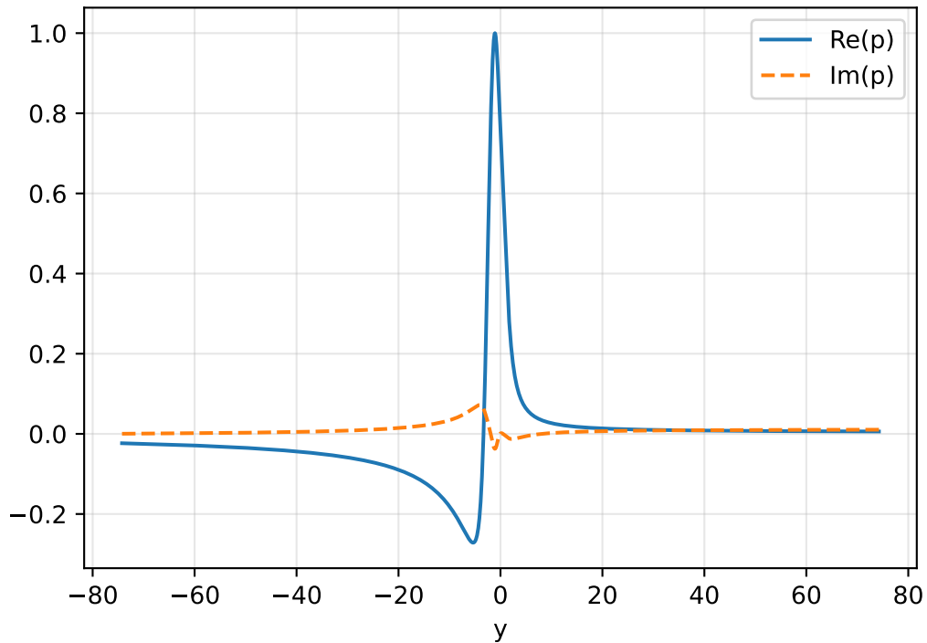
Mode PINN pour \alpha = 0.850
