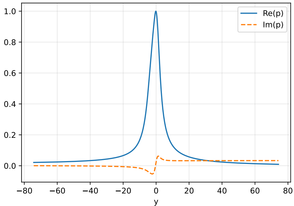
Mode PINN pour \alpha = 0.100
