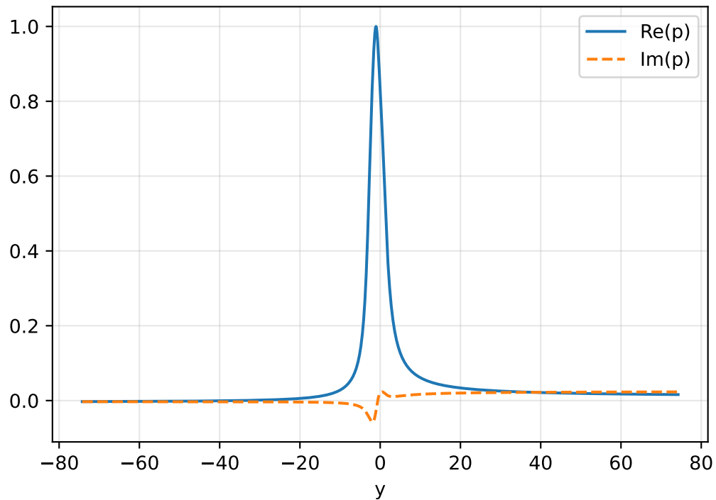
Mode PINN pour \alpha = 0.700
