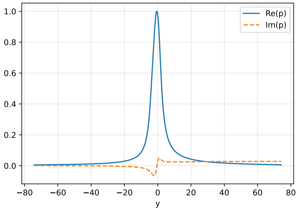
Mode PINN pour \alpha = 0.300
