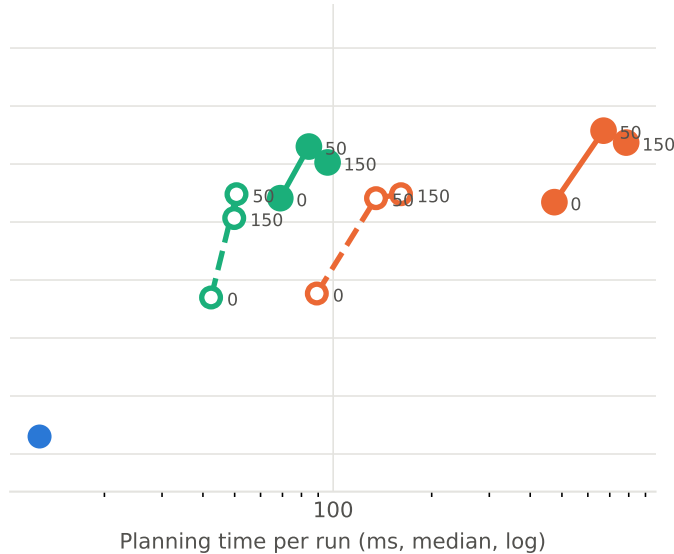
PRM (n = 146)
