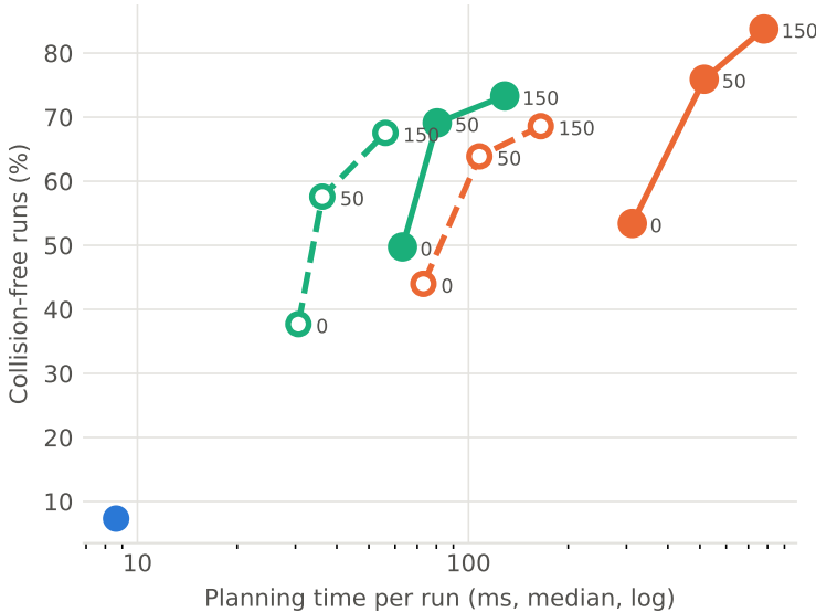
Voronoi (n = 191)
