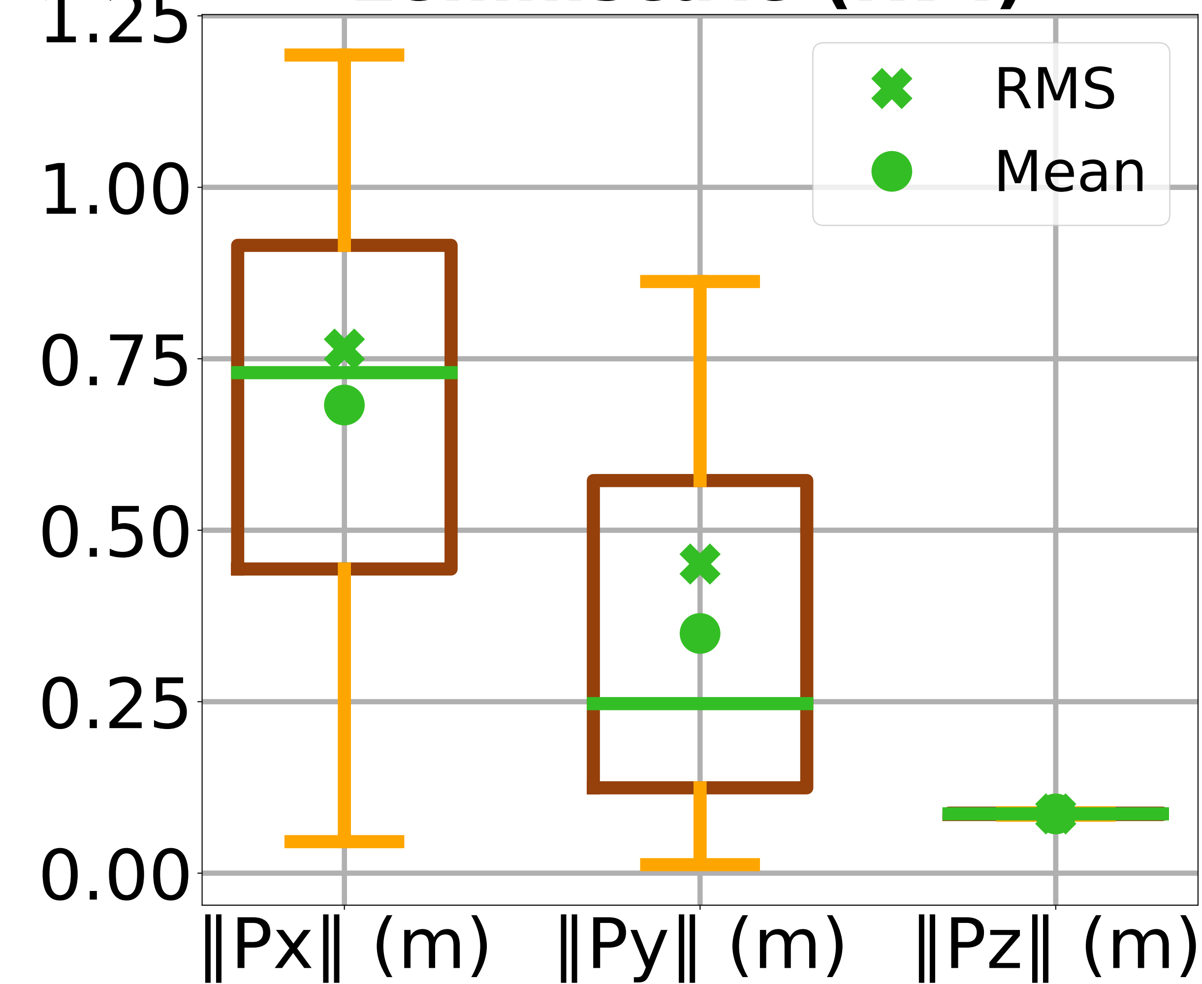
Lemniscate (NDI)
