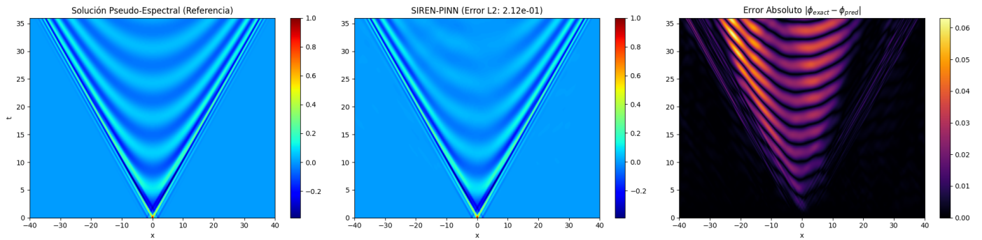
Figura 6: Mapa de error espacial de la PINN con activación SIREN. Los errores máximos se reducen respecto a la PINN vanilla, con una mejor captura de las oscilaciones.
