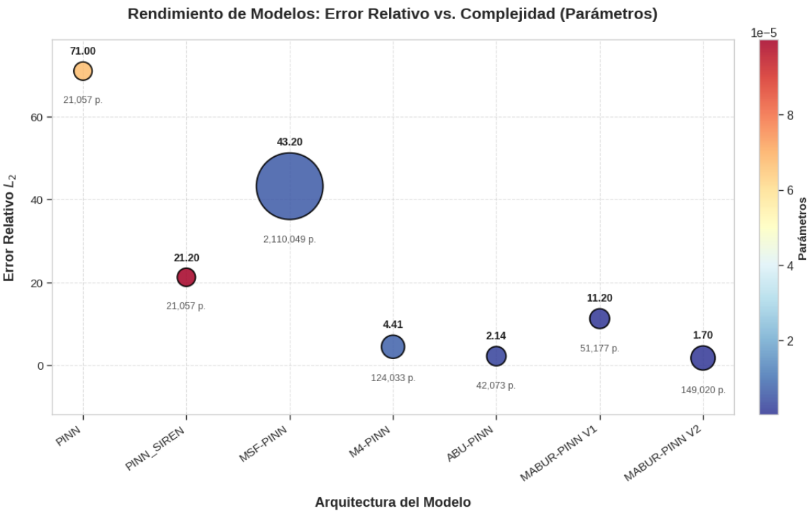
Figura 3: Diagrama comparativo de error relativo vs Complejidad (parámetros) para cada arquitectura.
