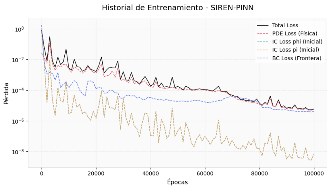
Figura 7: Historial de pérdidas para la PINN-SIREN. La pérdida asociada a las condiciones de iniciales de posición alcanza valores bajos ( \sim 10^{-8} ).
