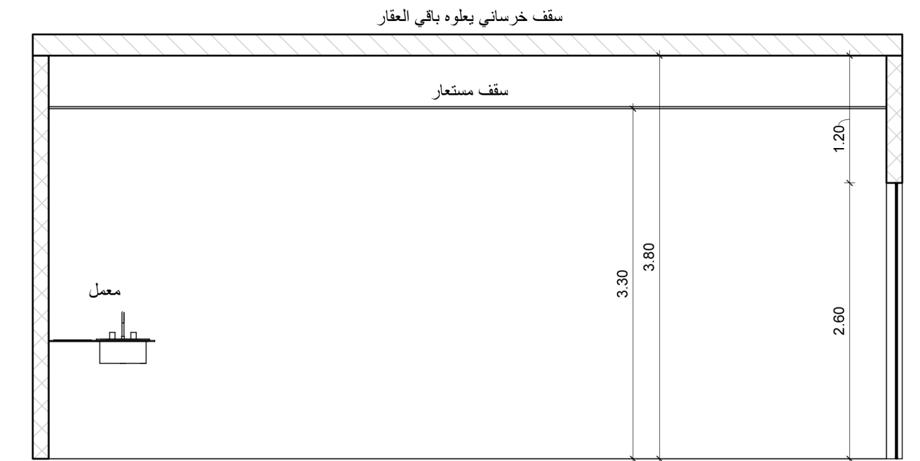
4 قطاع رأسي 1 : 50
