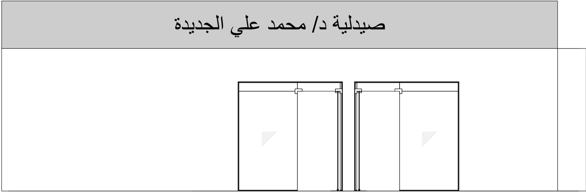
1 واجهة أمامية 1 : 50
