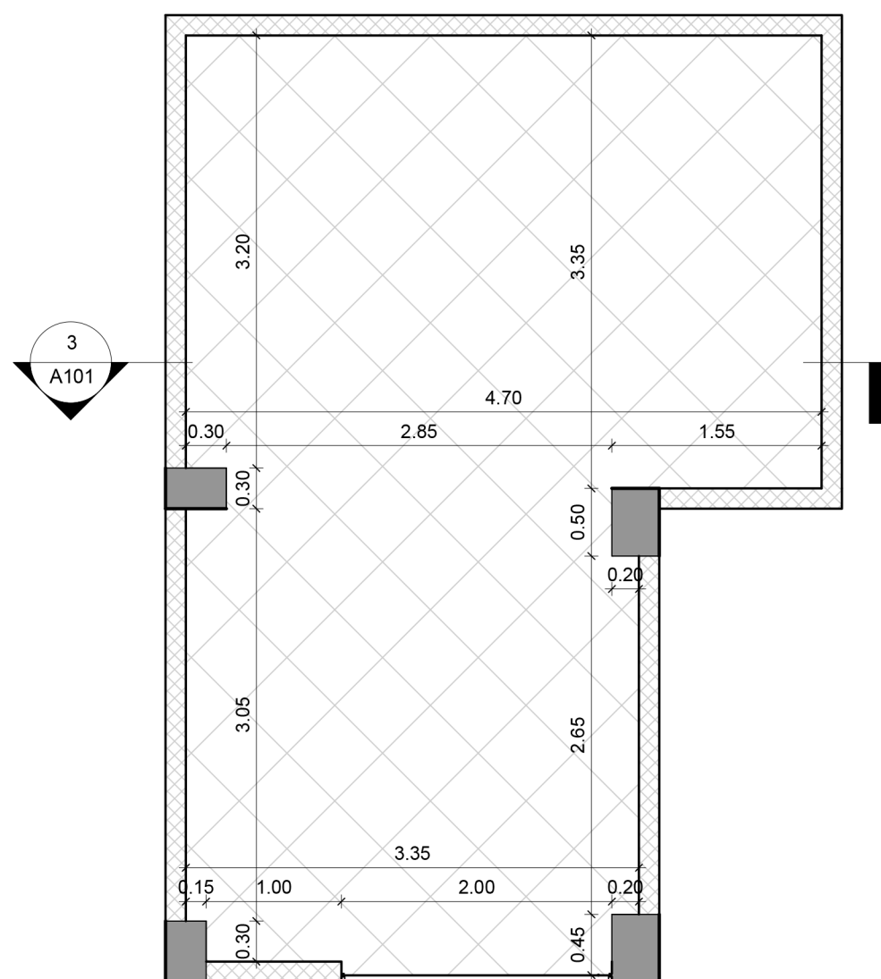
1 مسقط أفقي 1 : 50
