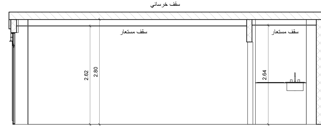
5 قطاع رأسي 1 : 50
