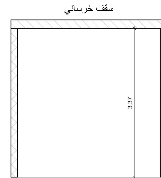
3 قطاع رأسي 1 : 50
