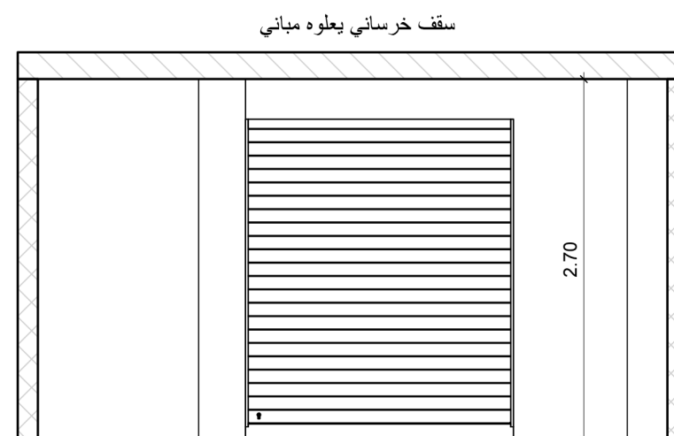
3 قطاع رأسي 1 : 50
