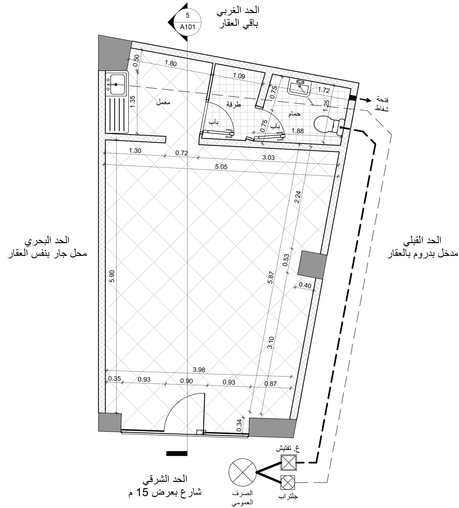
1 مسقط أفقي 1 : 50
