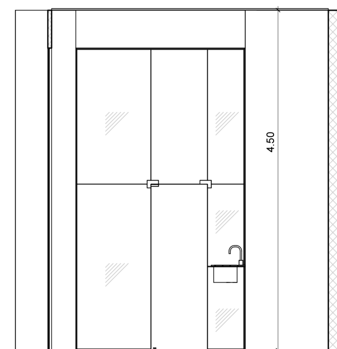
3 قطاع رأسي 1 : 50
