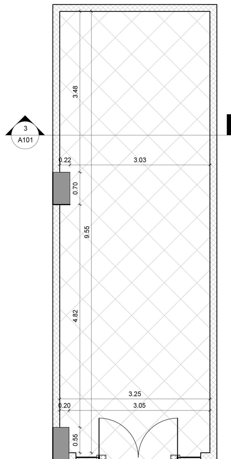
1 مسقط أفقي 1 : 50
