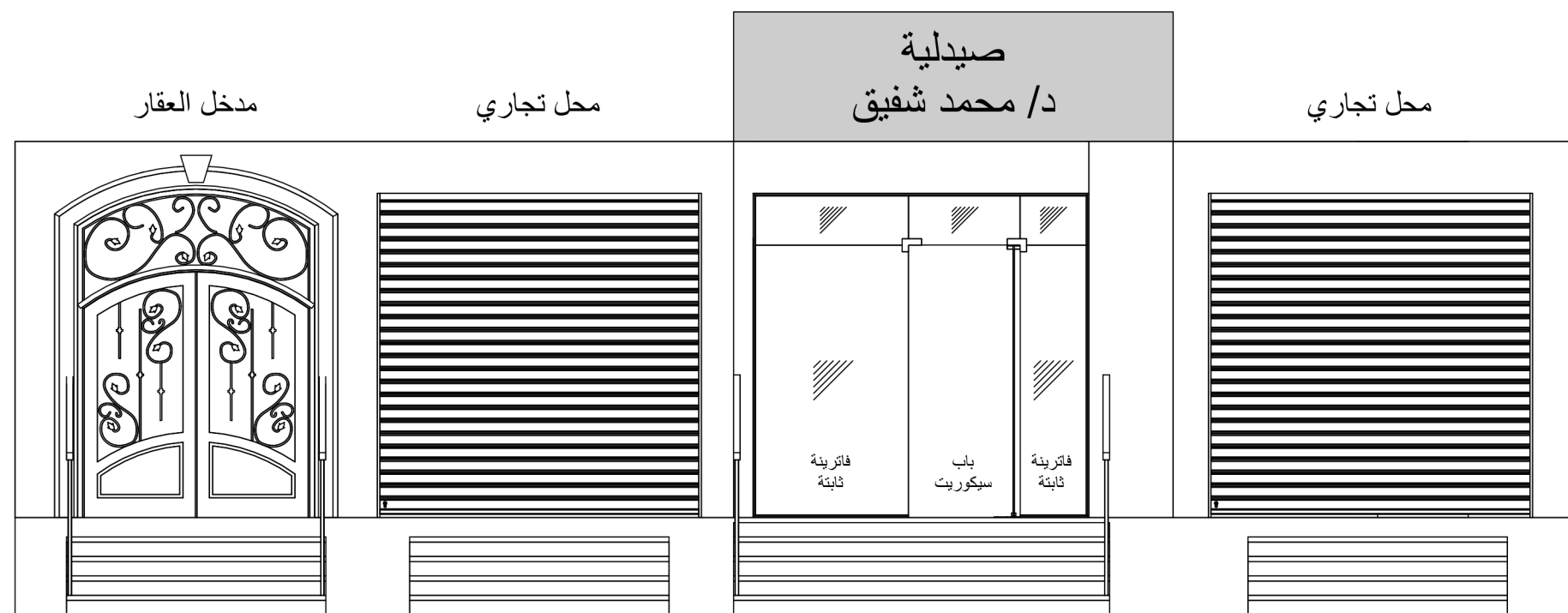
2 واجهة أمامية 1 : 50
