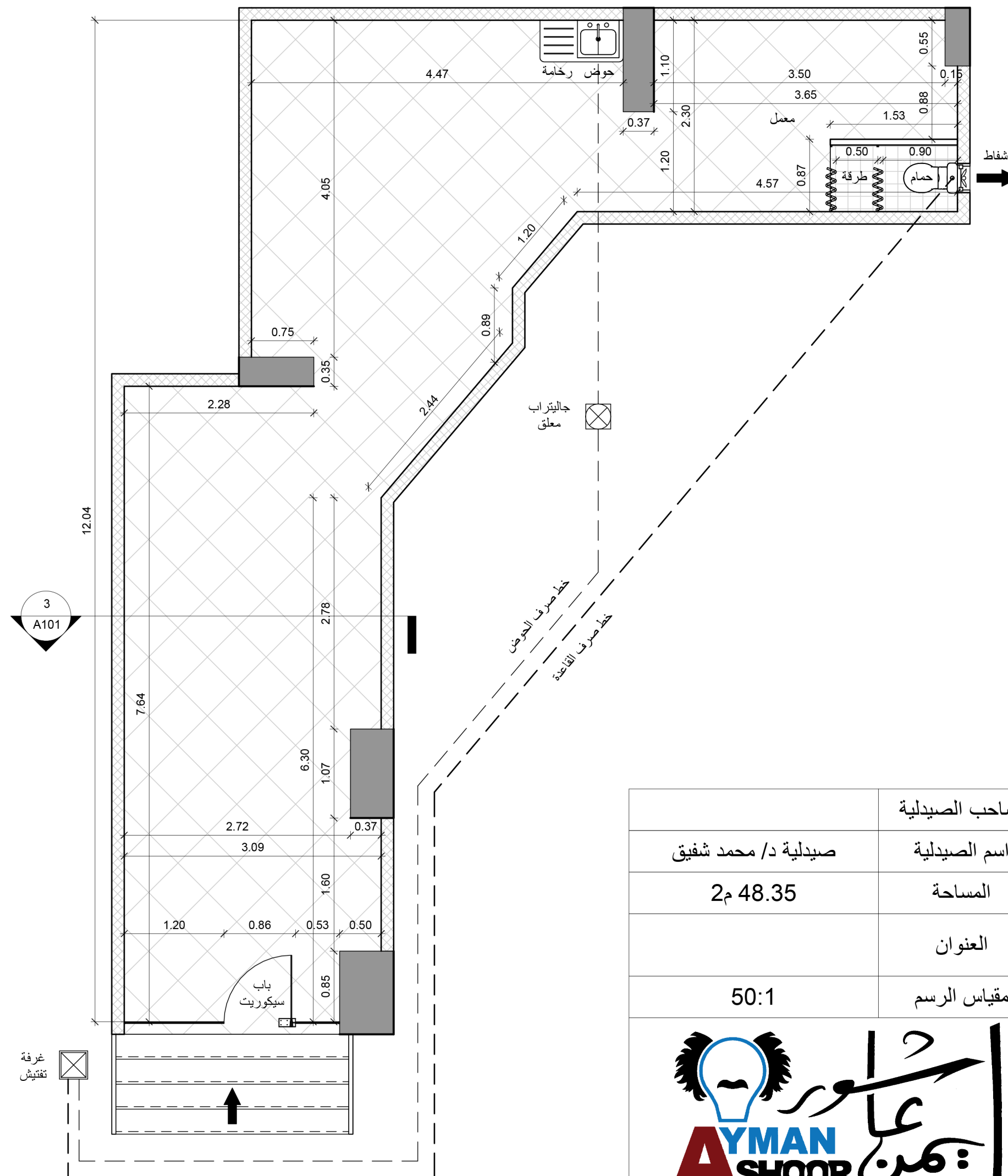
1 مسقط أفقي 1 : 50
