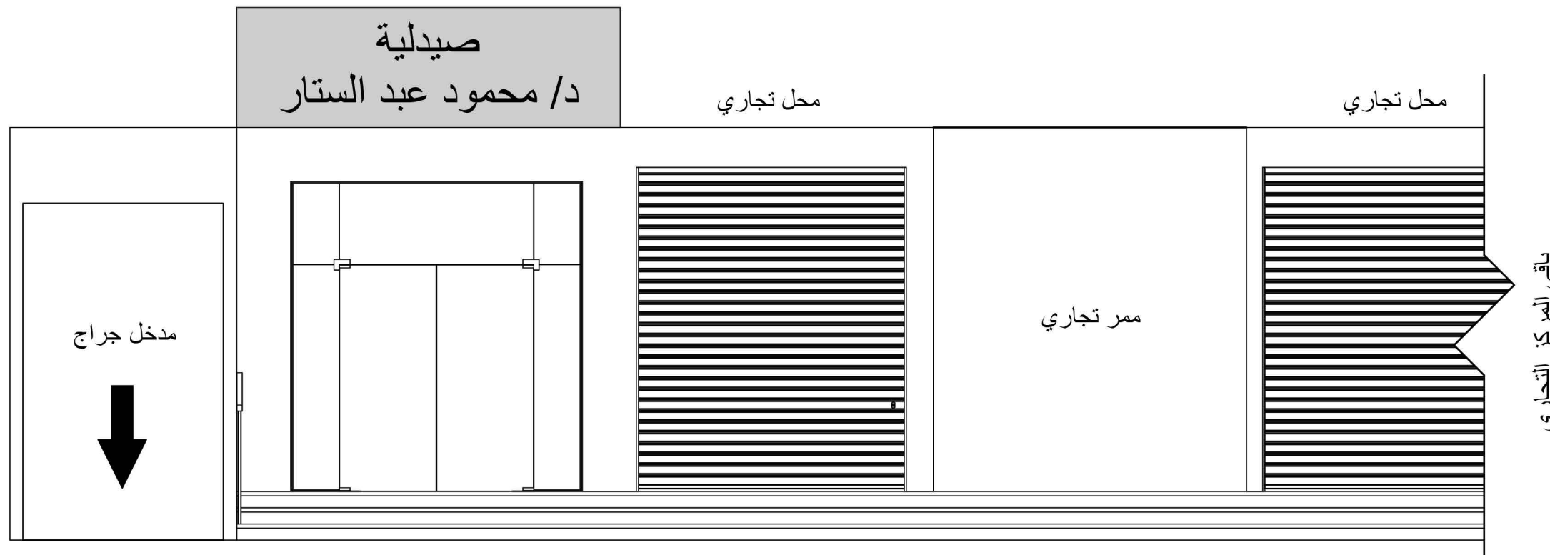
2 واجهة أمامية 1 : 50
