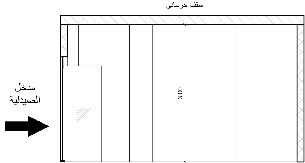
3 قطاع رأسي 1 : 50
