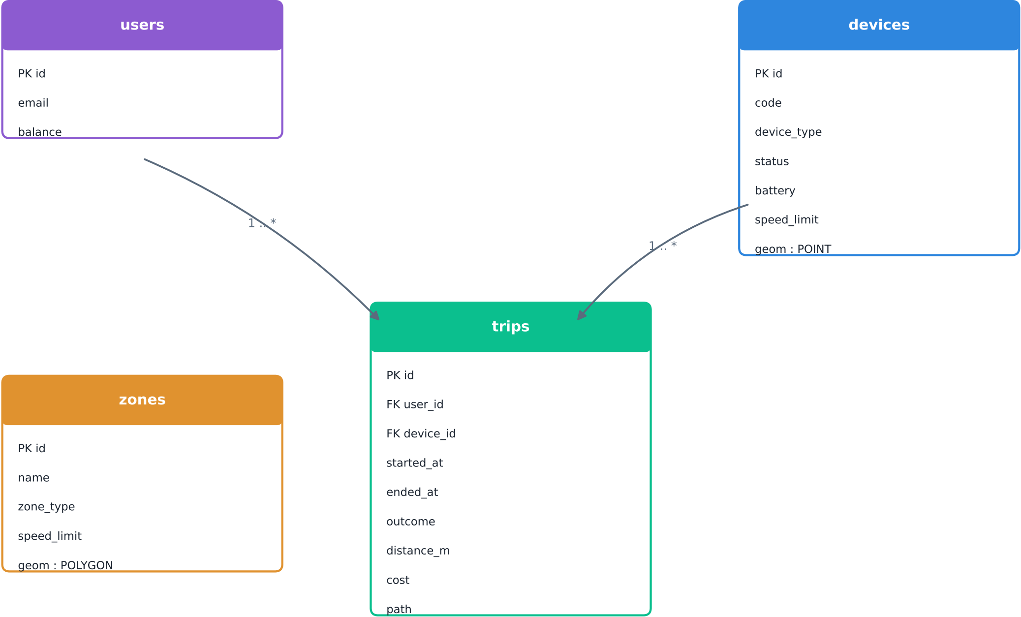
Рис. 2 — Схема базы данных (ER)
