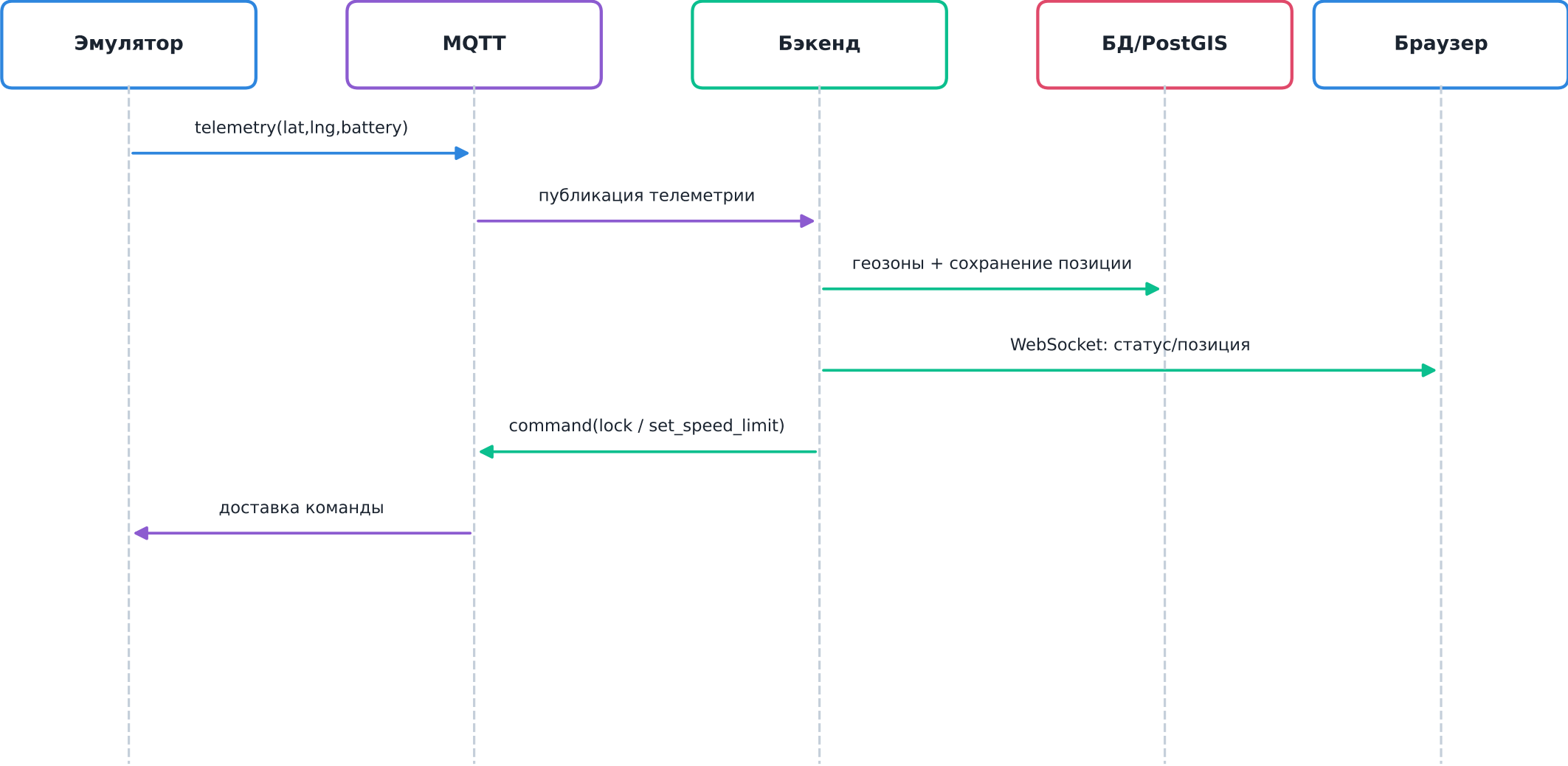
Рис. 4 — Обработка телеметрии (диаграмма последовательности)
