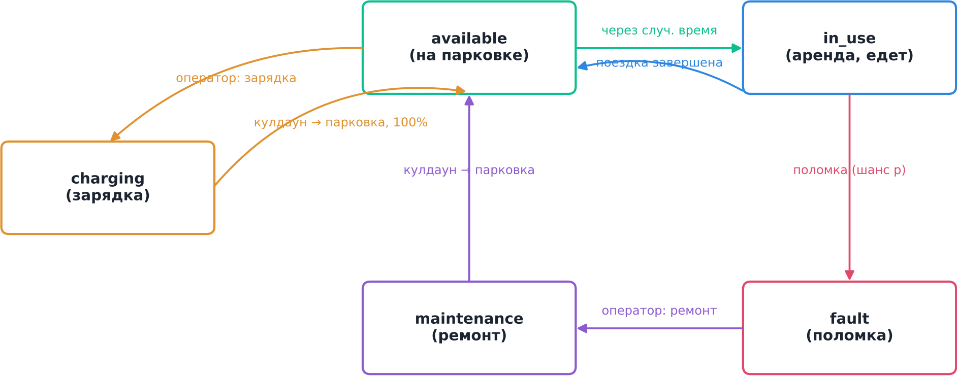
Рис. 3 — Жизненный цикл самоката (диаграмма состояний)
