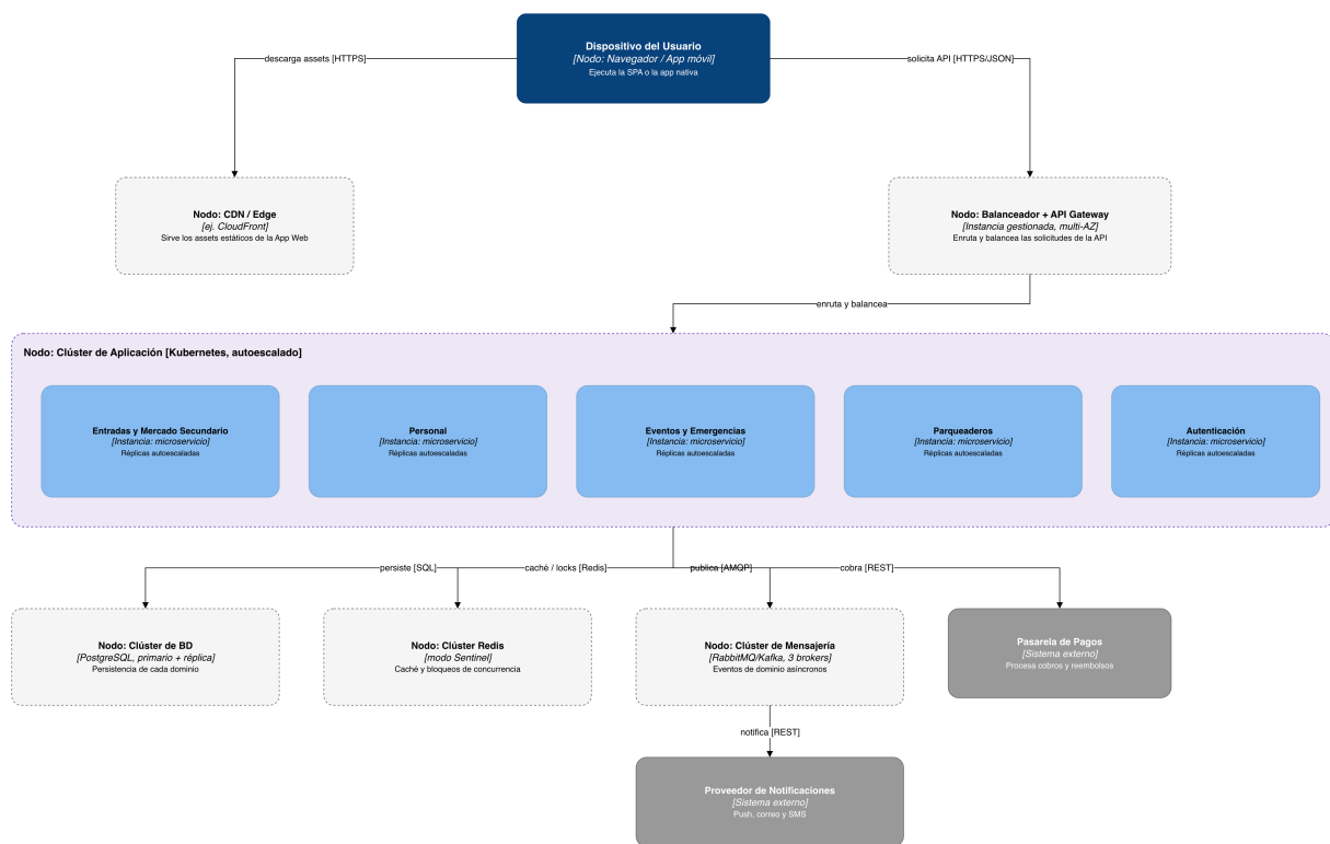
Figure 5: Diagrama de despliegue — ambiente de producción (modelo C4).
