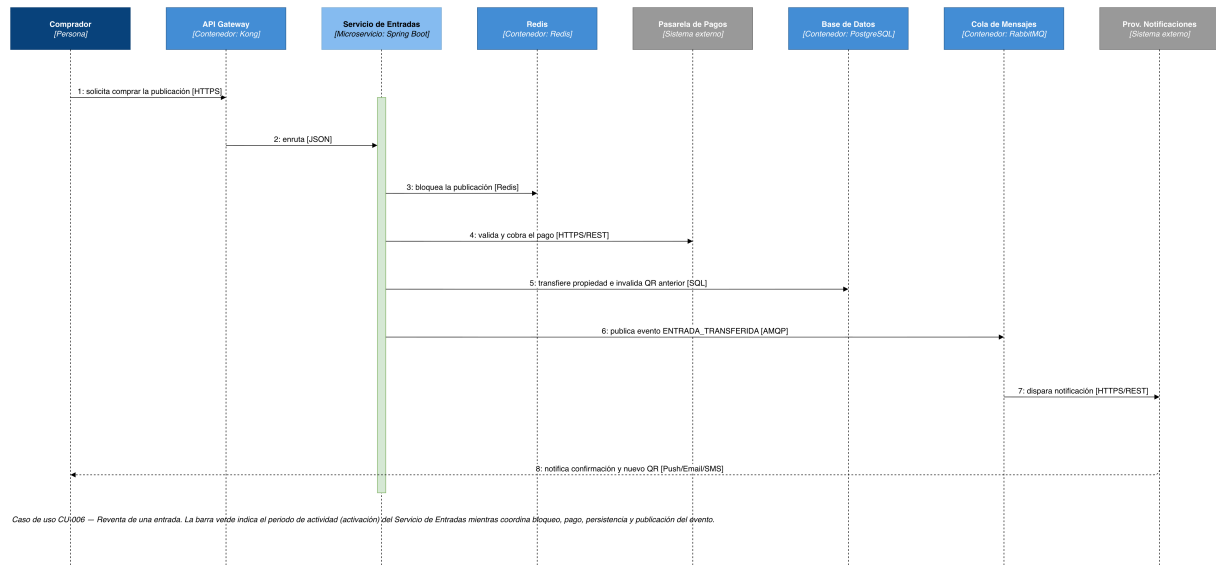
Figure 4: Diagrama de secuencia — reventa de una entrada (CU-006).
