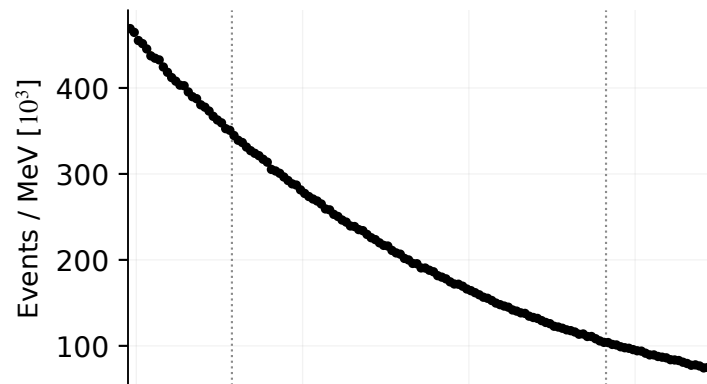
2016: 117 MeV
