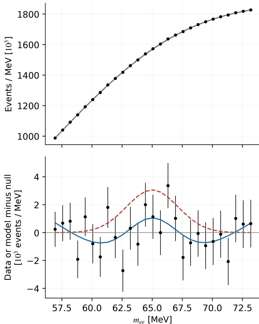
2021: 65 MeV
