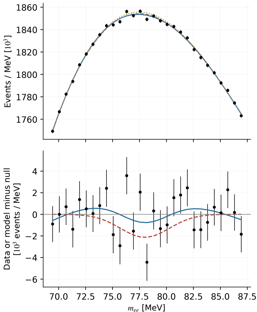
2021: 78 MeV
