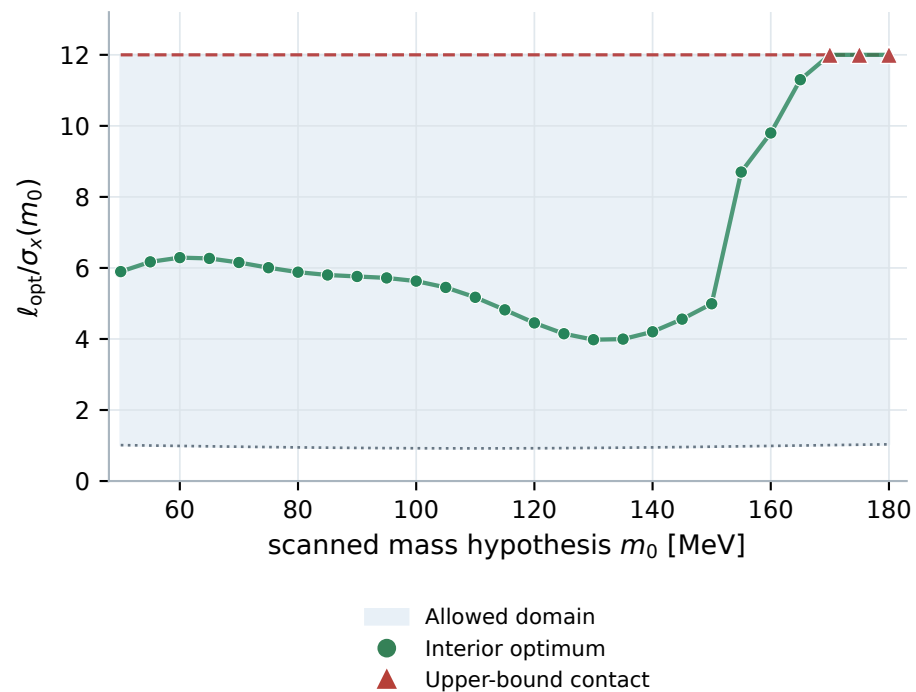
(d) Interior and boundary optima
