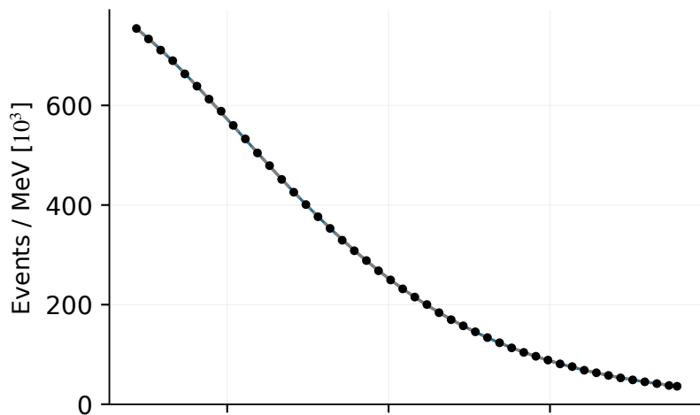
2015: 51 MeV
