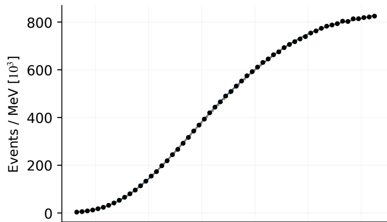
2015: 21 MeV
