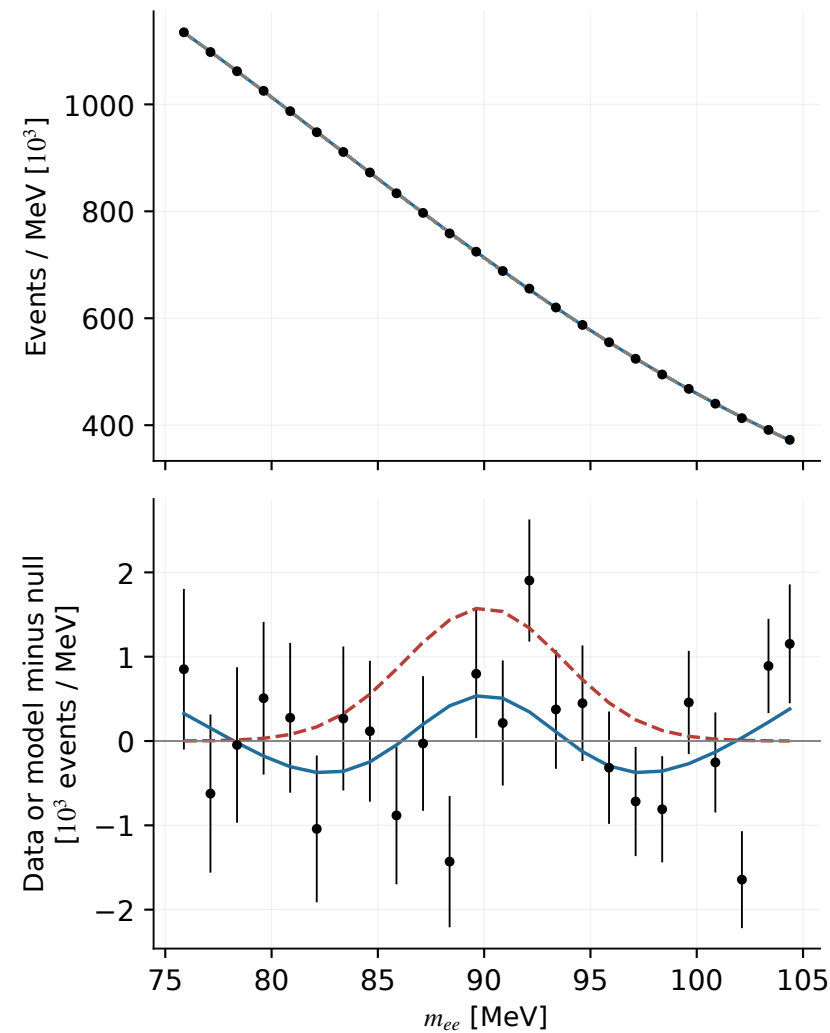
2016: 90 MeV
