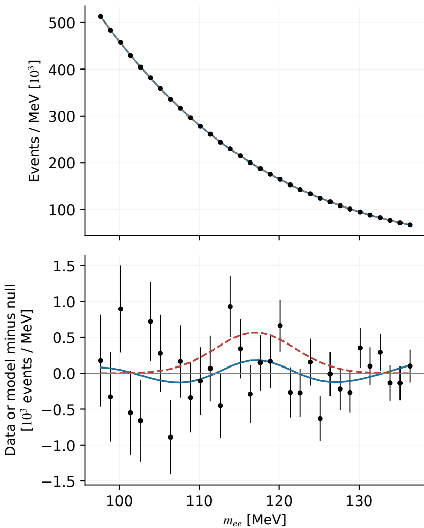
2016: 117 MeV
