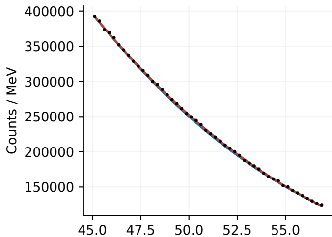
2015: 51 MeV
