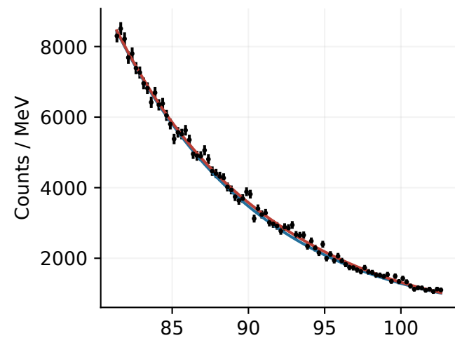
2015: 92 MeV
