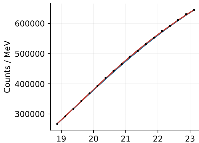
2015: 21 MeV
