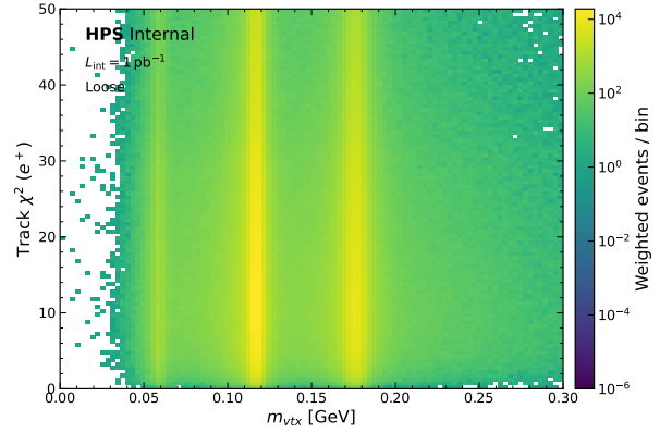
(d) Mass vs. positron \chi^2 (signal).
