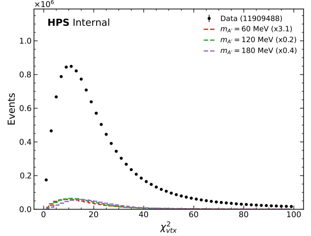
(b) Vertex-fit \chi^2 .
