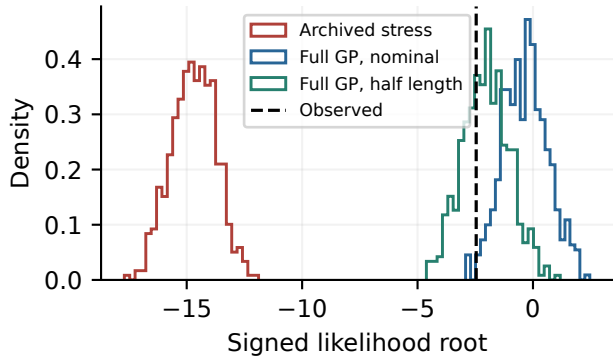
76 MeV
