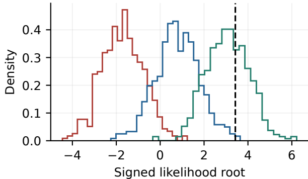
90 MeV
