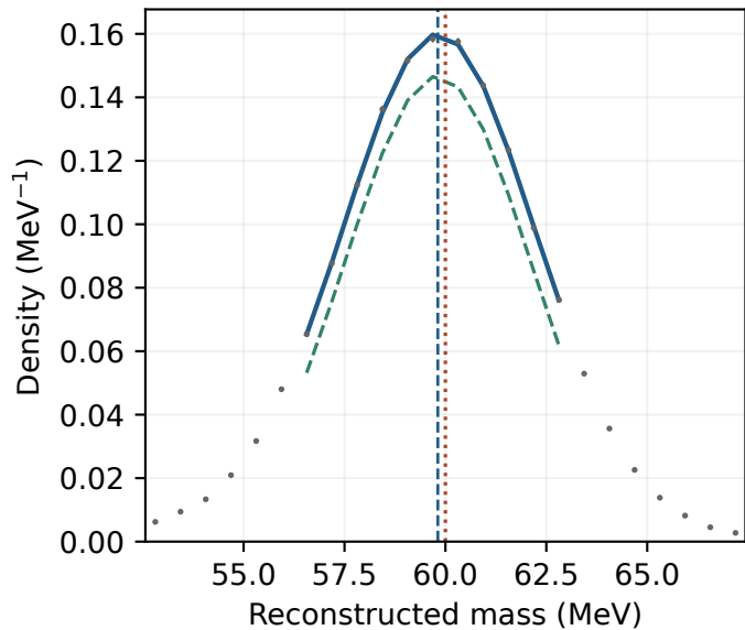
60 MeV: core shift -0.188 MeV
