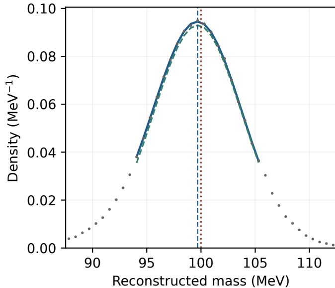
100 MeV: core shift -0.309 MeV
