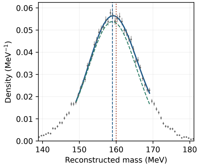
160 MeV: core shift -1.017 MeV
