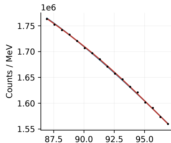
2021: 92 MeV
