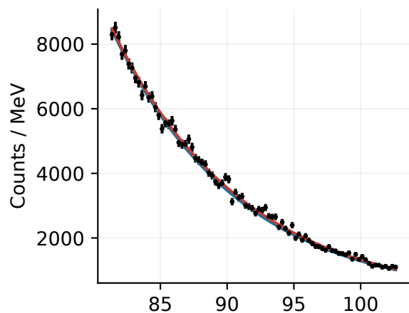
2015: 92 MeV
