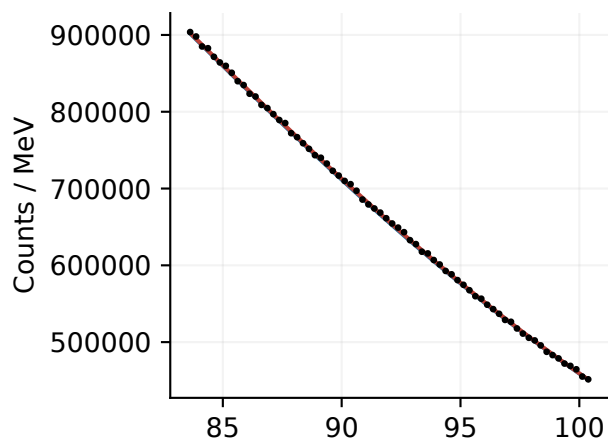
2016: 92 MeV
