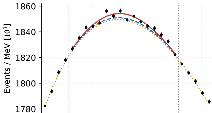
2021: 78 MeV
