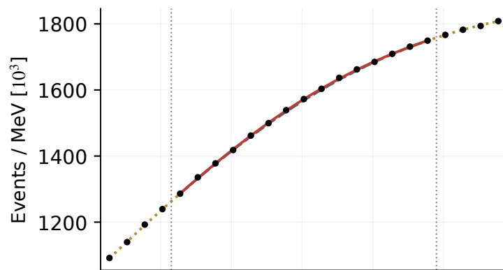
2021: 65 MeV
