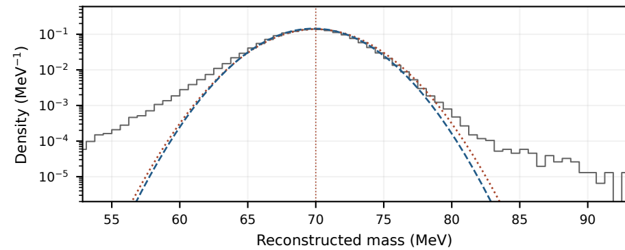
70 MeV; N = 245,676
