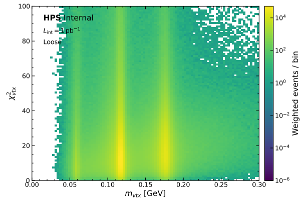
(f) Mass vs. vertex \chi^2 (signal).
