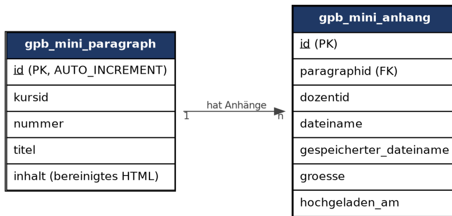
Abbildung 2 ERD
