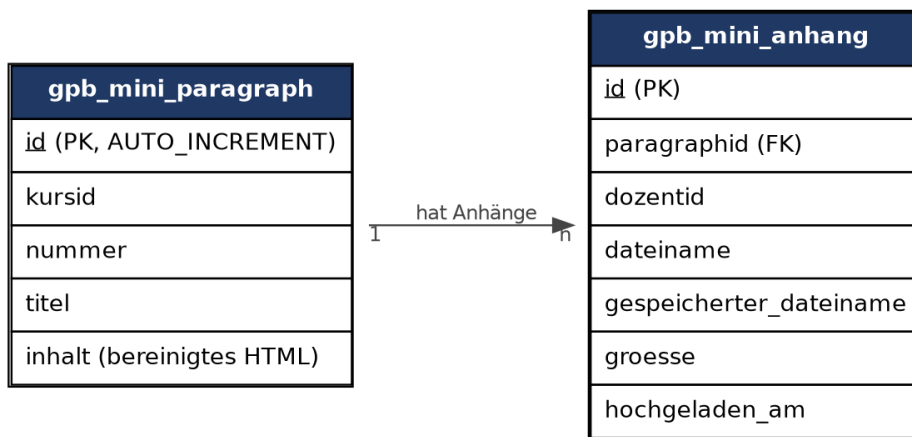
Abbildung 2 ERD
