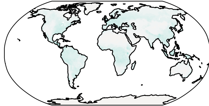
b) TRENDY
