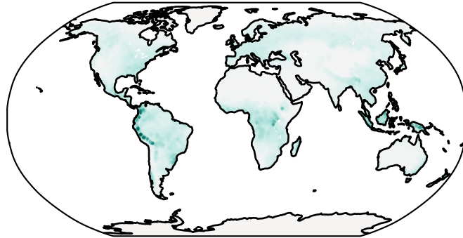
a) CMIP6
