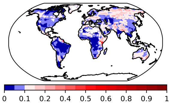
NCC
