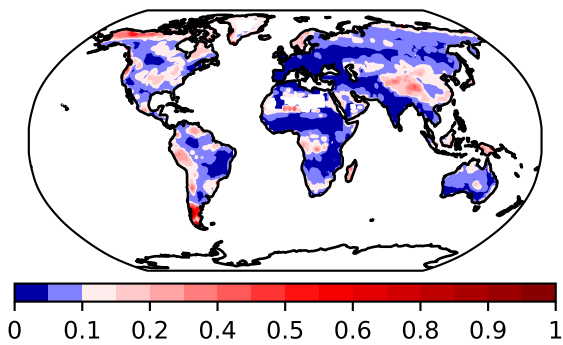
CSIRO
