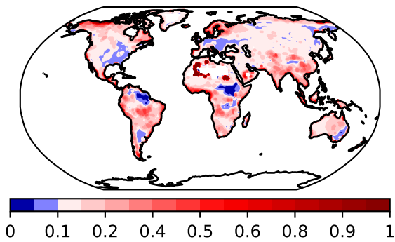
MPI
