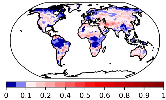
NOAA
