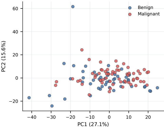
PCA Projection
