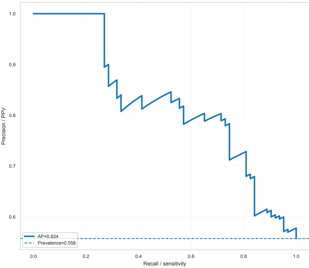
Precision-Recall Curve ADC_Post1_Post2_Pre | elasticnet_then_mrrmr_auto_k_no_smote | SVM_RBF
