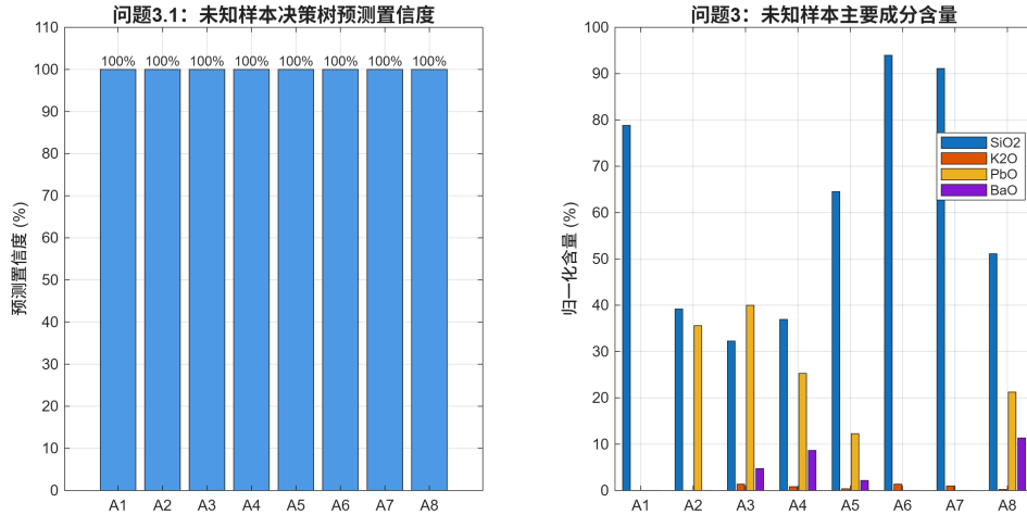
图 5: 未知样本预测置信度（左）与主要成分含量对比（右）
