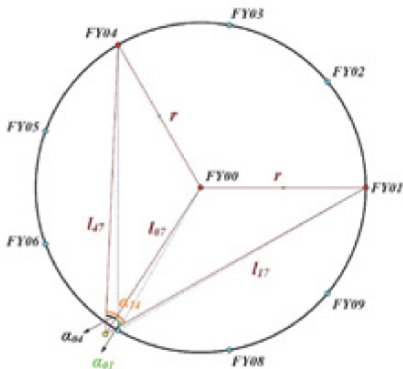
图 1: 三架无人机无源定位示意图
