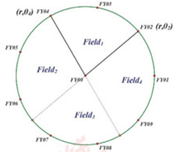
图 3: 正弦定理求解坐标的局限性
