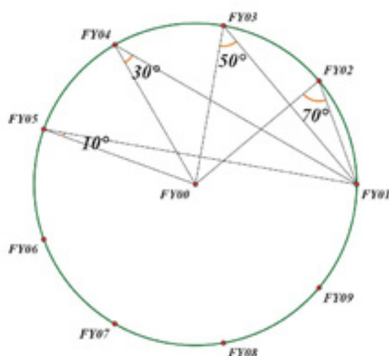
图 6: 标准位置角度 (1)
