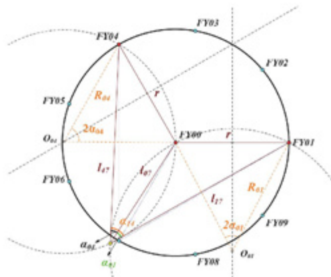
图 4: 等角对等边示意图
