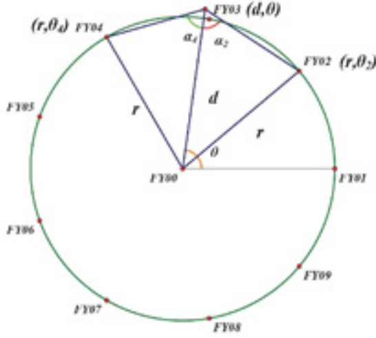
图 2: 正弦定理求解坐标
