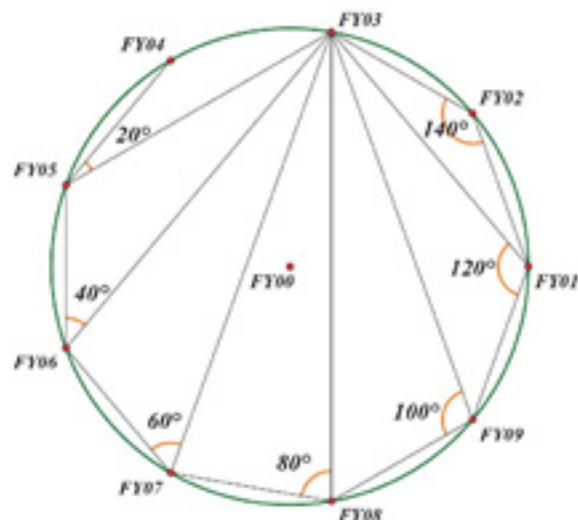
图 7: 标准位置角度 (2)
