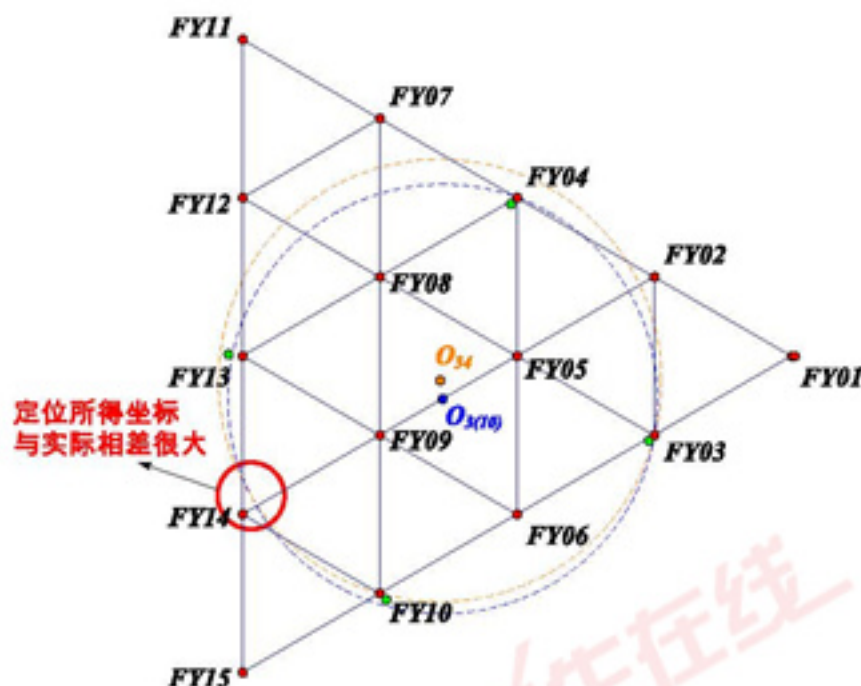
图 17: 四点共圆情况示意
