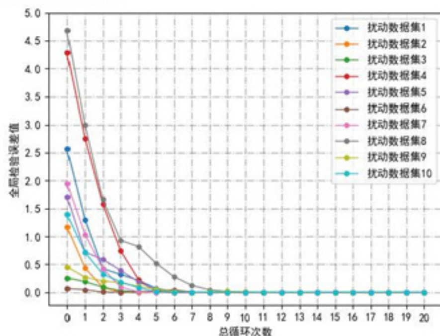
图 28 十组数据集的全局检验误差值
