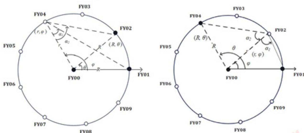
图 2-3 主动机与被动机排布的两种情况
