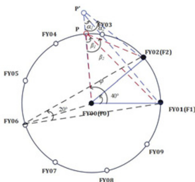
图 7 排布方式 1 的被动机位置
