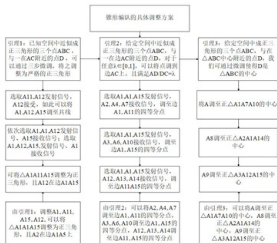
图 24 锥形编队调节的流程图
