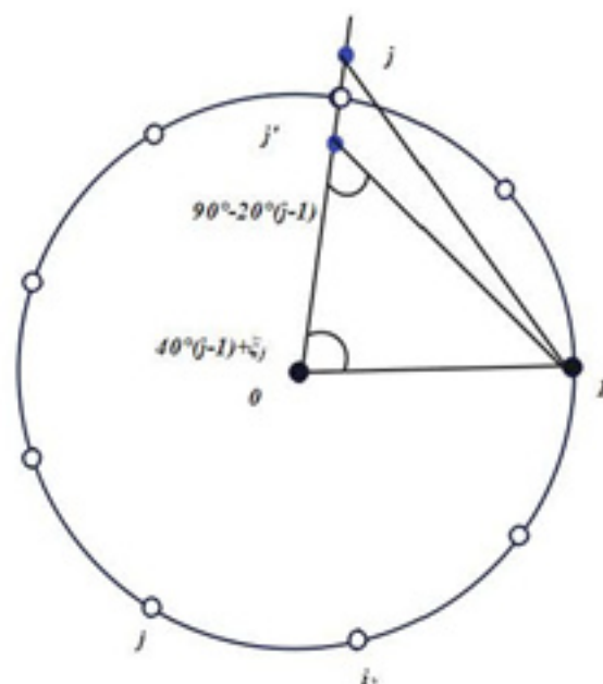
图 12 预处理证明示意图
