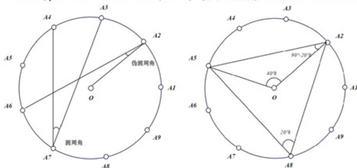
图 8-9 角的定义与引理的证明
