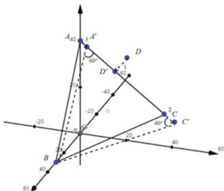
图 20 引理 1 的调整方案
