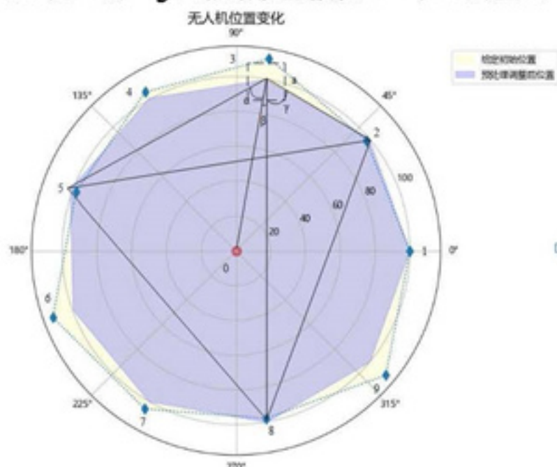
图 14 方案一预处理后的调整图示
