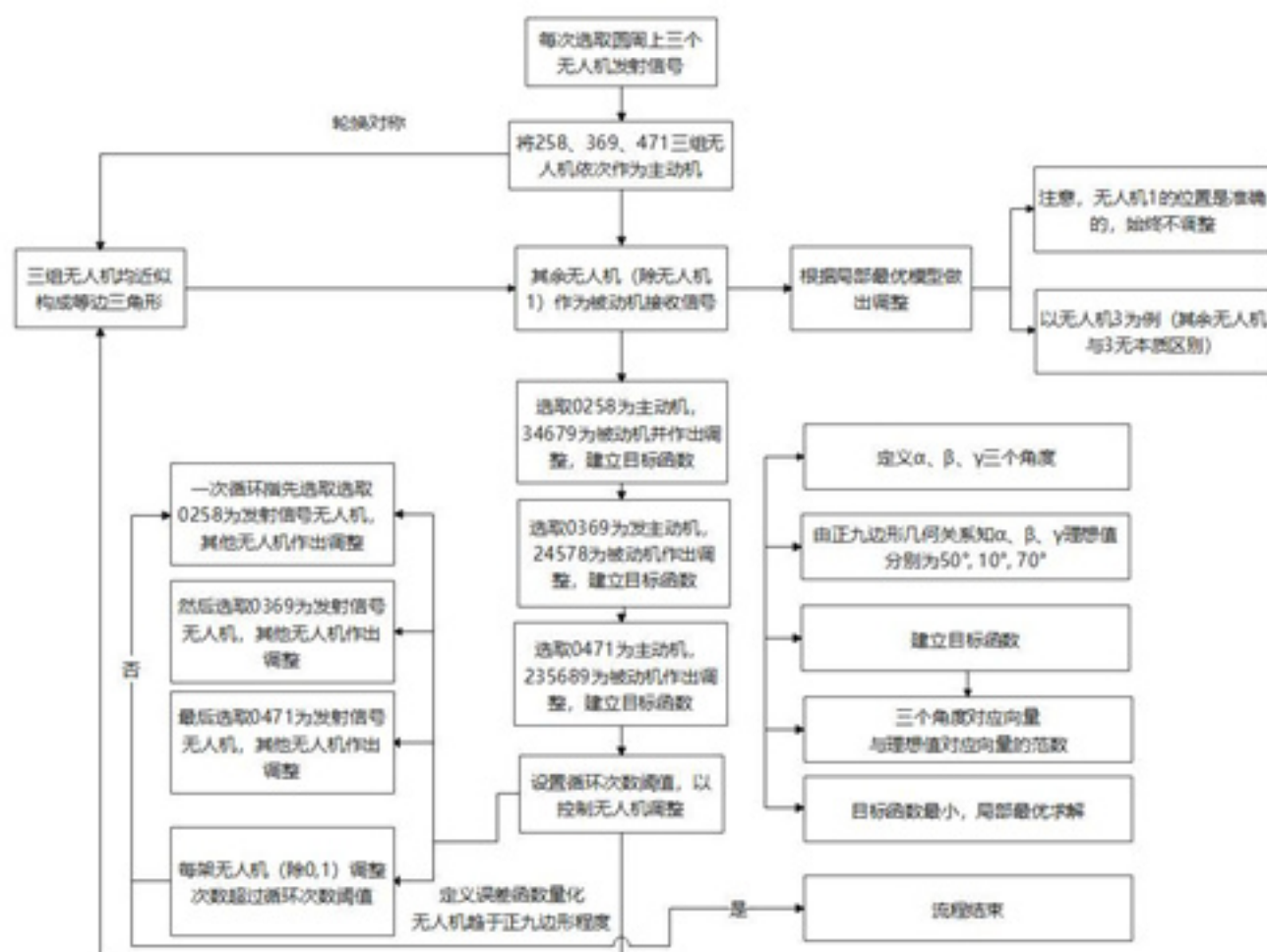
图 15 方案一对应的流程图
