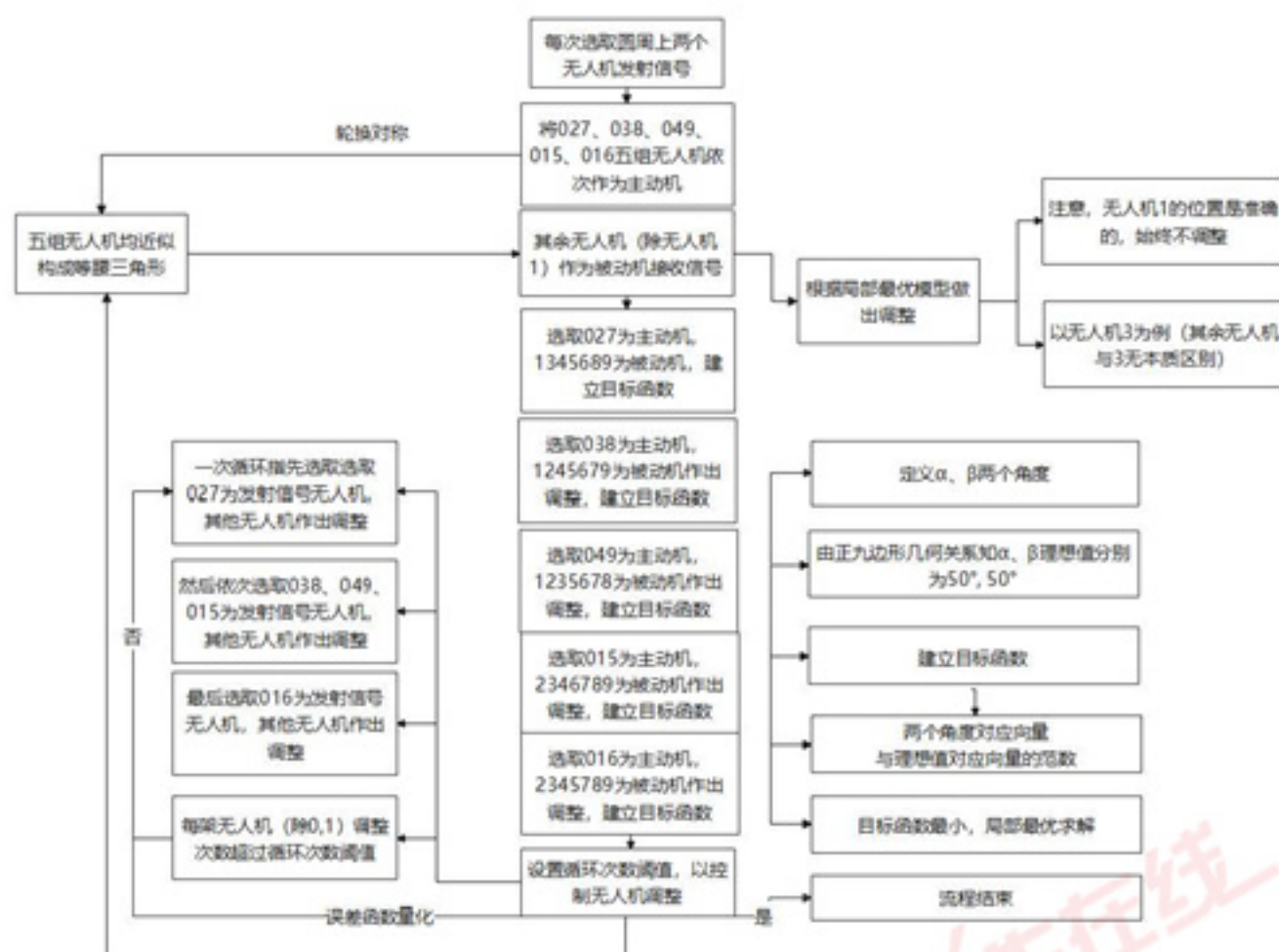
图 17 方案二对应的流程图
