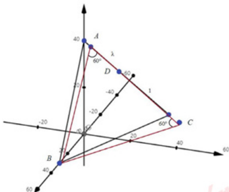
图 21 引理 2 的几何关系
