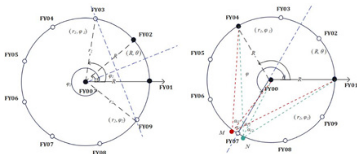
图 4-5 解的几何分布及特殊情况
