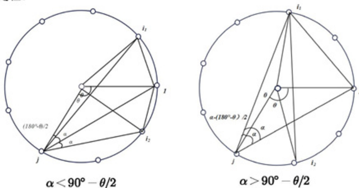
图 10-11 主动机的两种分布情况
