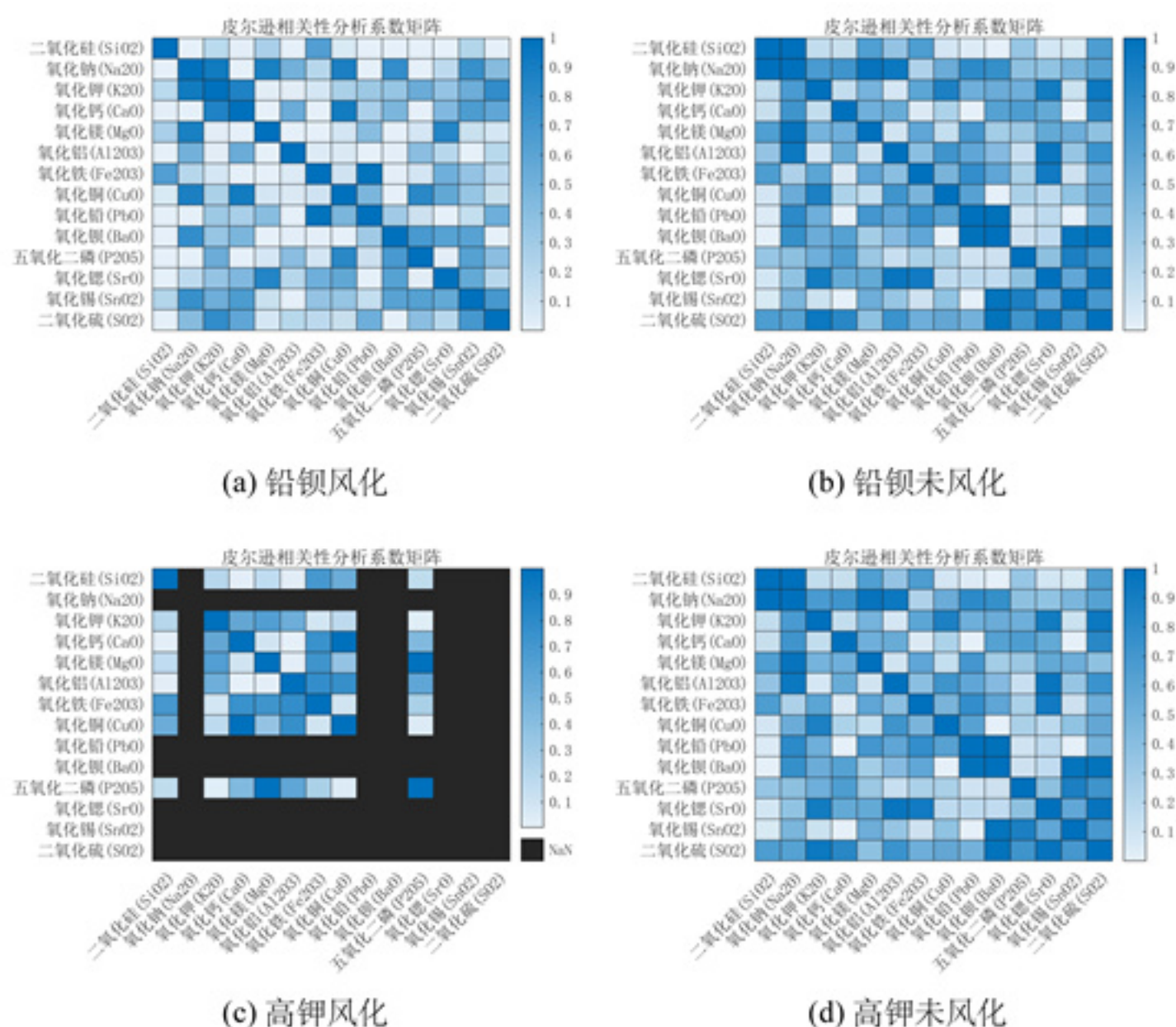
图 6 四类相关系数矩阵
