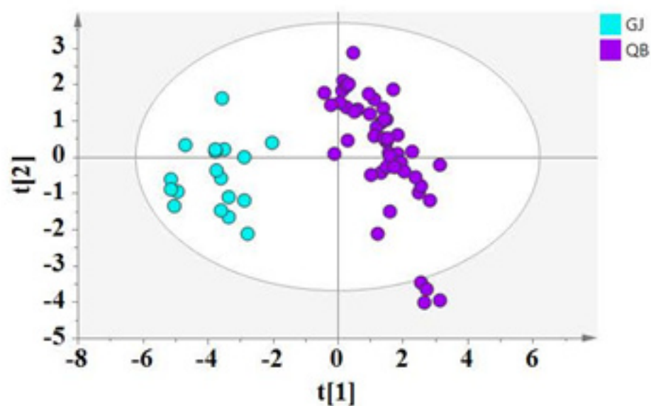
图 10：偏最小二乘判别分析结果
