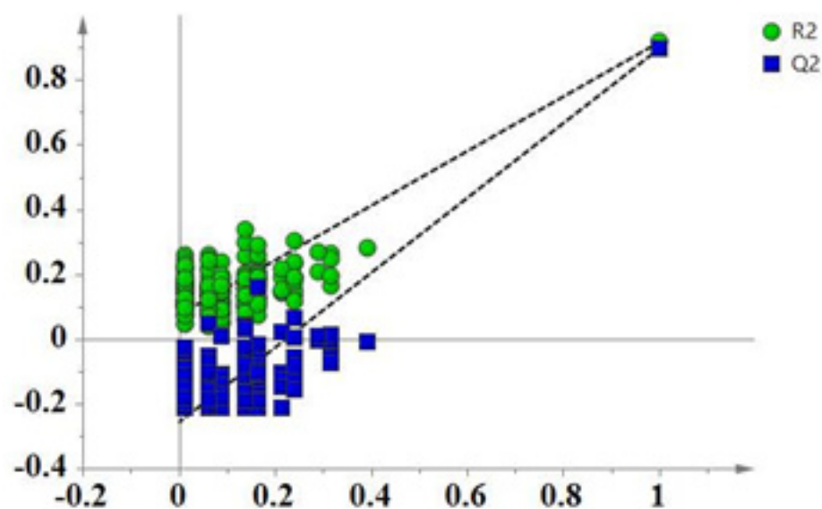
图 11：偏最小二乘判别分析模型验证
