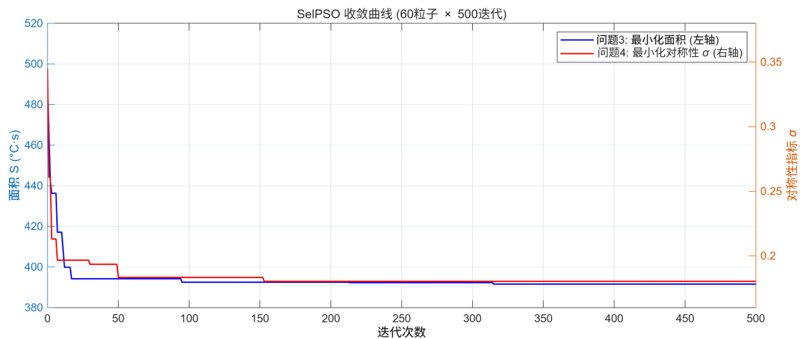
图 4: SelPSO 收敛曲线 (60 粒子 \times 500 迭代)
