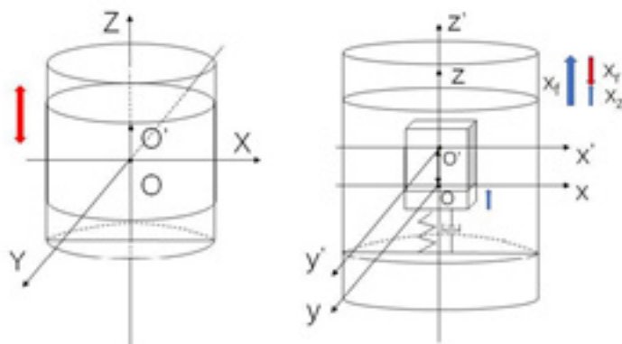
图 1 大地坐标系和固体坐标系示意图
