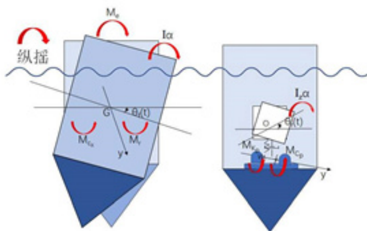
图 10 纵摇运动受力分析示意图
