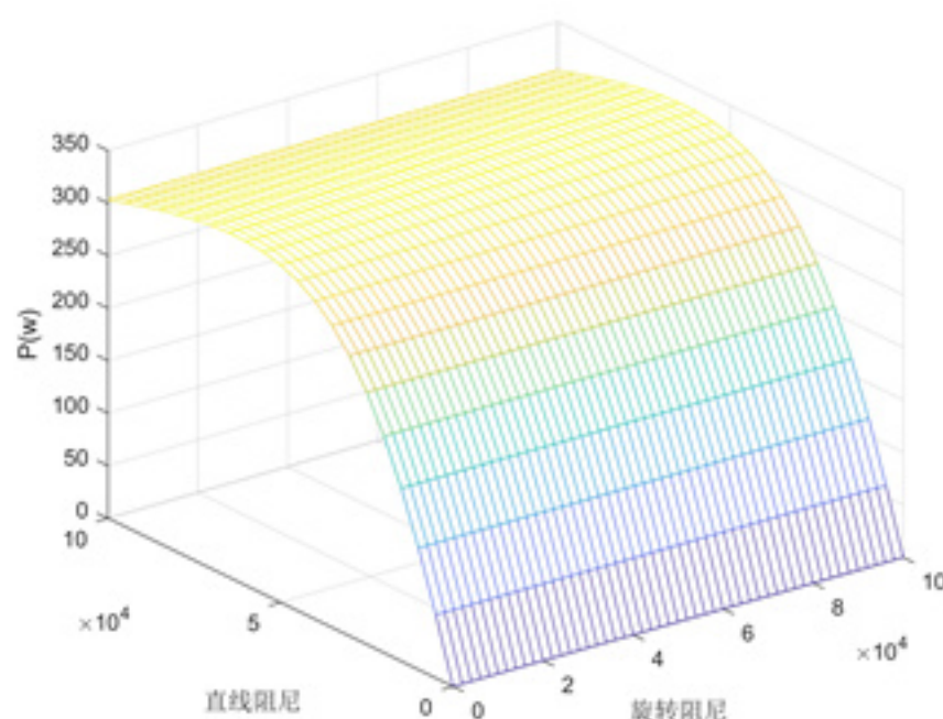
图 13 不同阻尼系数下的功率分布图
