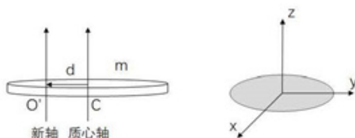
图9 平行移轴和垂直轴定理示意图
