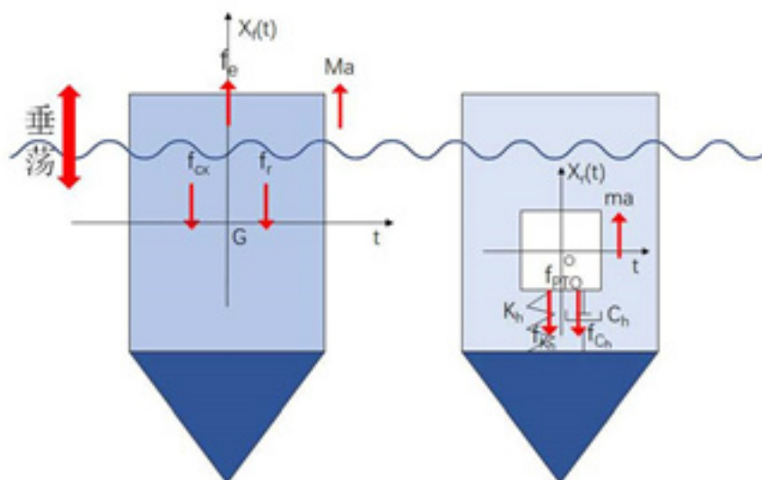
图2 垂荡运动受力分析示意图
