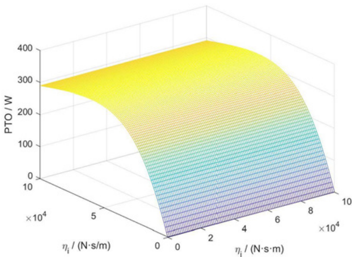
图 12 PTO 关于 \eta_i 和 \eta_j 的全局遍历图
