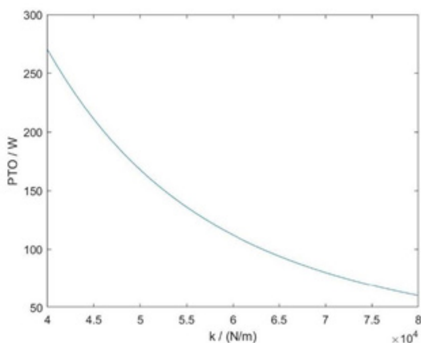
图 18 弹簧刚度的稳定性分析图
