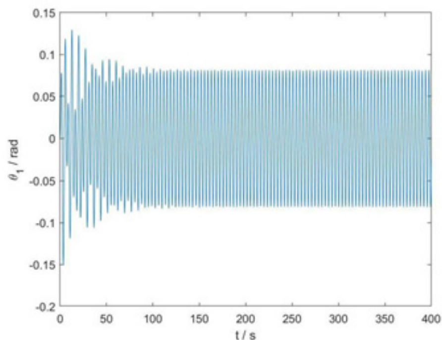
图 10 \theta_1 关于时间的变化
