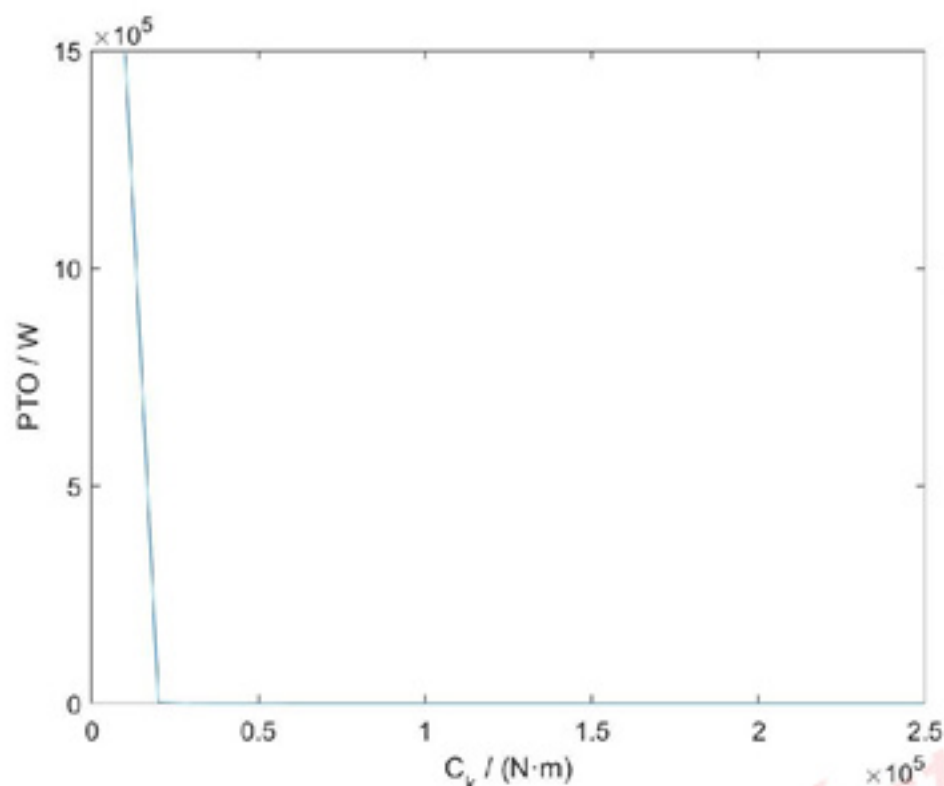
图 17 扭转弹簧刚度的稳定性分析图
