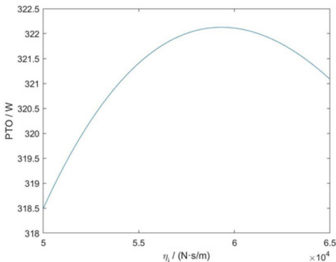
图 13 PTO 关于 \eta_i 的局部遍历图
