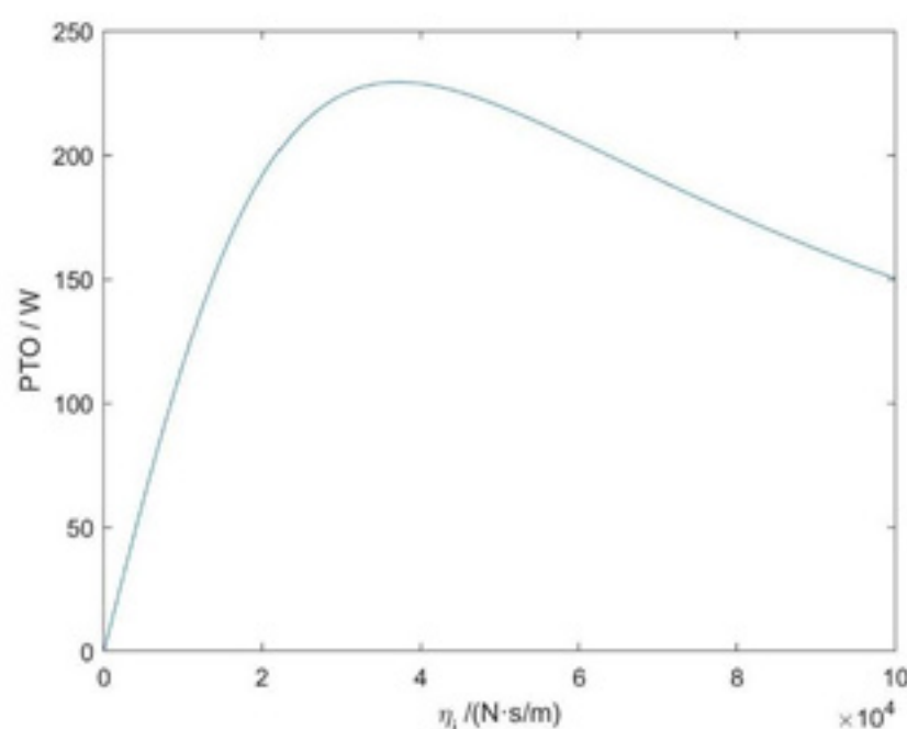
图 3 PTO 关于 \eta_i 的函数图 1
