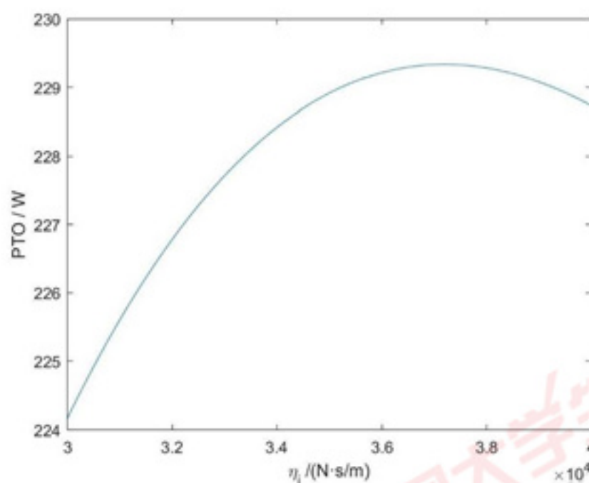
图 4 PTO 关于 \eta_i 的函数图 2
