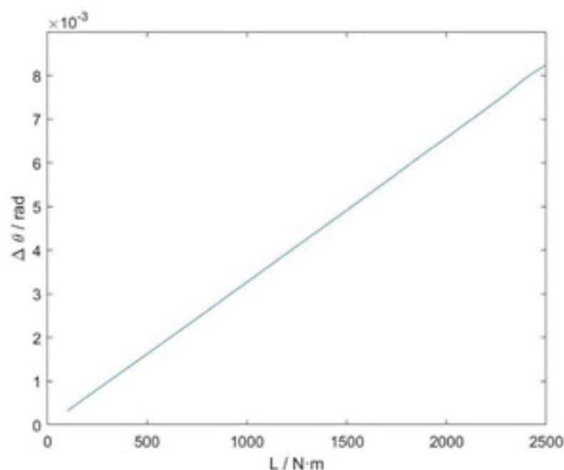
图 16 波浪激励力矩的稳定性分析图
