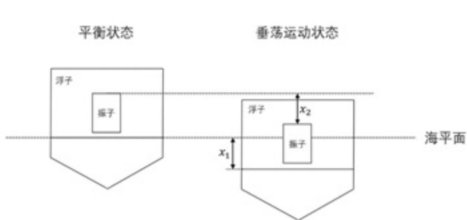
图 1 浮子坐标示意图
