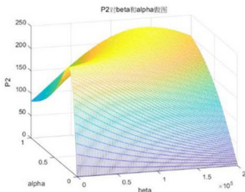
图8 P 对 \beta 和 \alpha 作图
