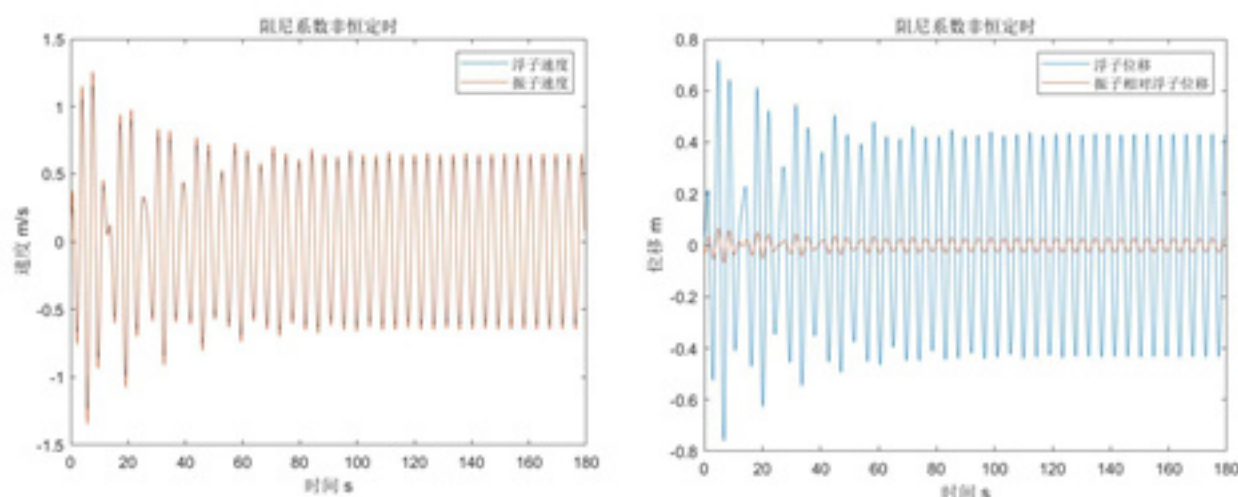
图 5 阻尼系数非恒定时结果曲线
