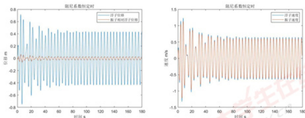
图4 阻尼系数恒定时结果曲线
