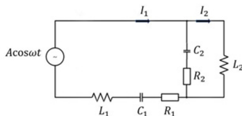
图 6 力电比拟等效电路图
