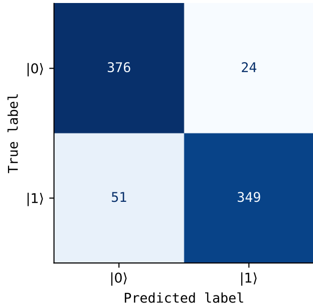
MLP
