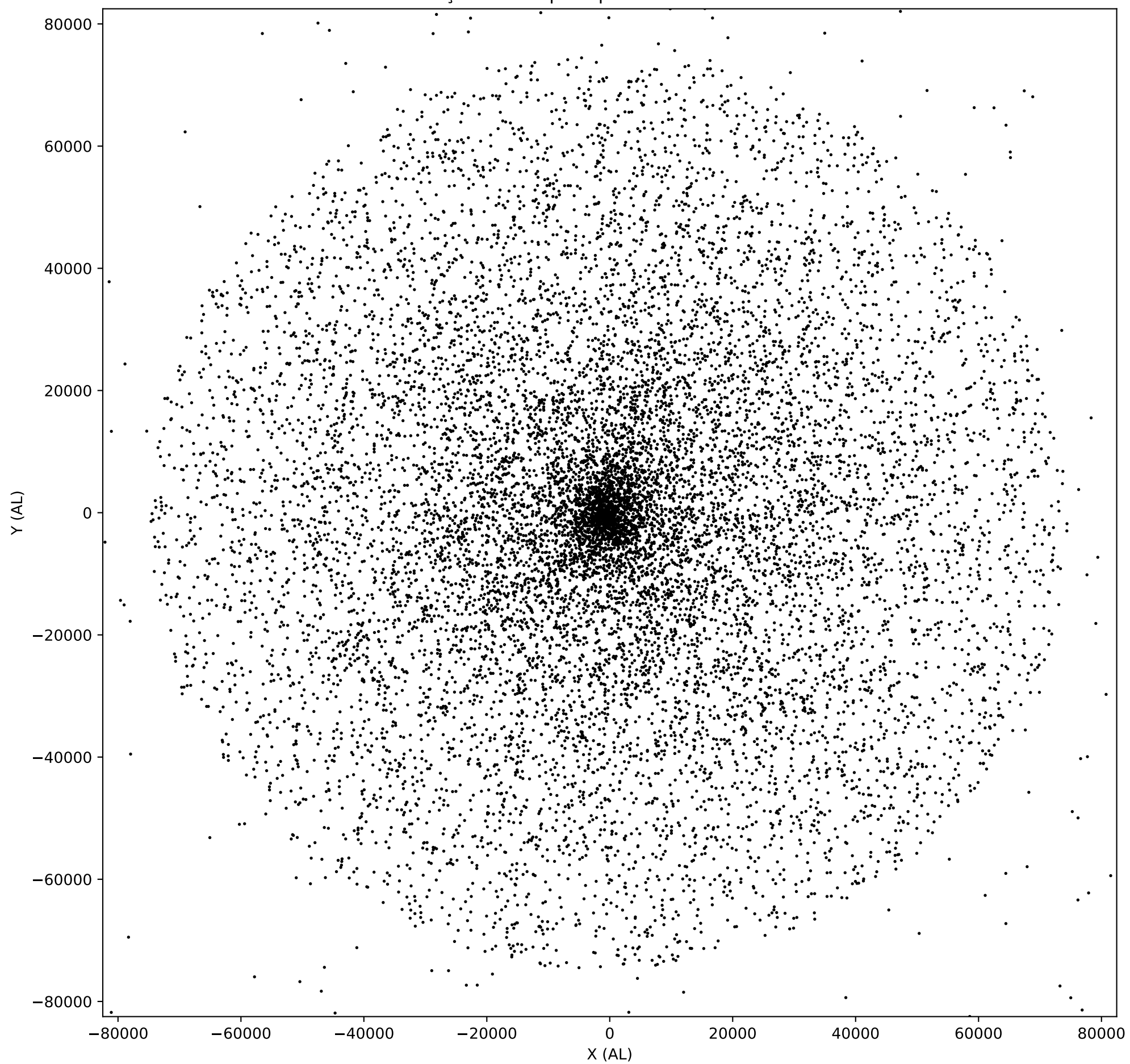
Distribuição dos corpos apos 29000.000000 milenios
