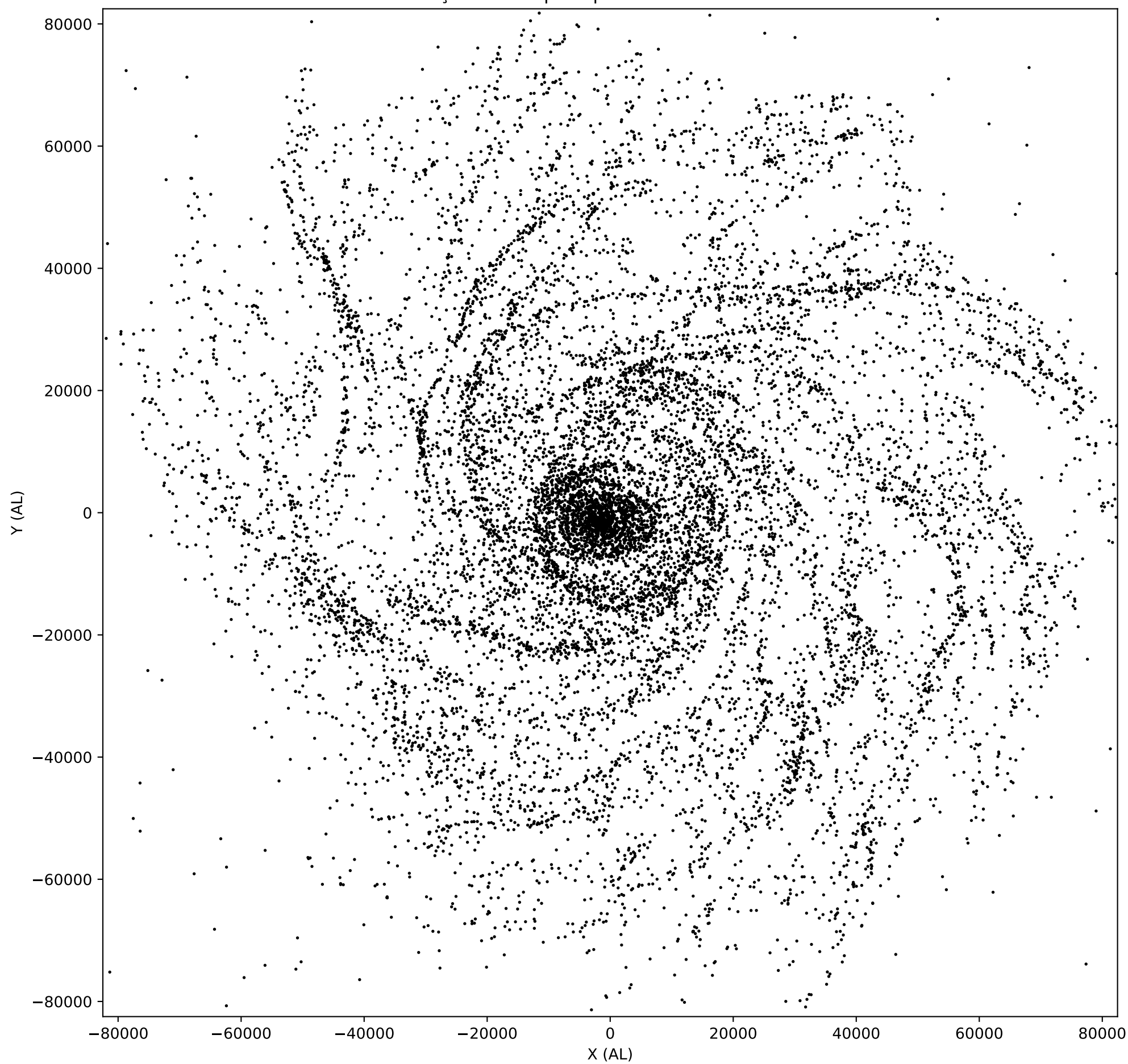
Distribuição dos corpos apos 291200.000000 milenios
