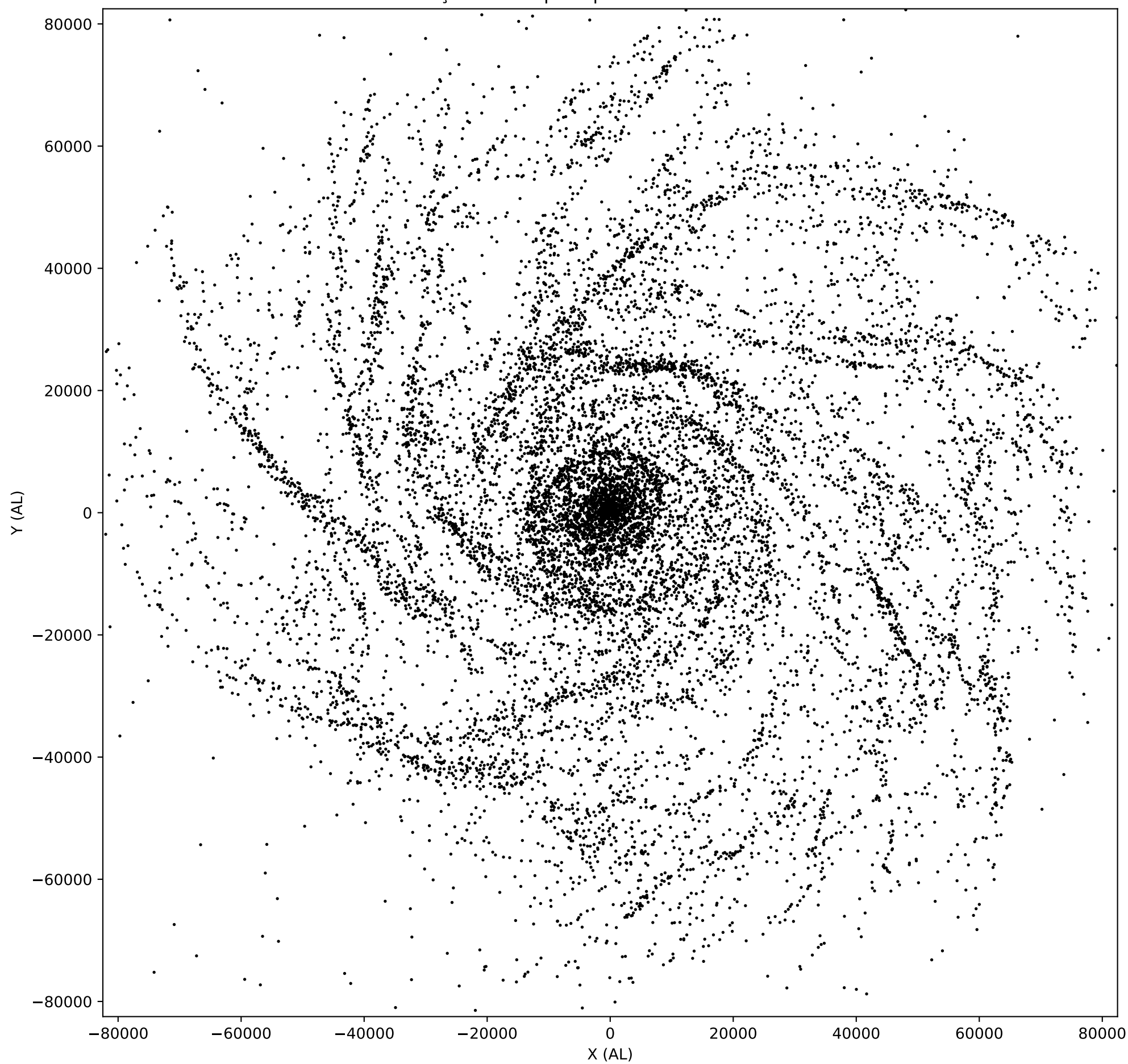
Distribuição dos corpos apos 320300.000000 milenios
