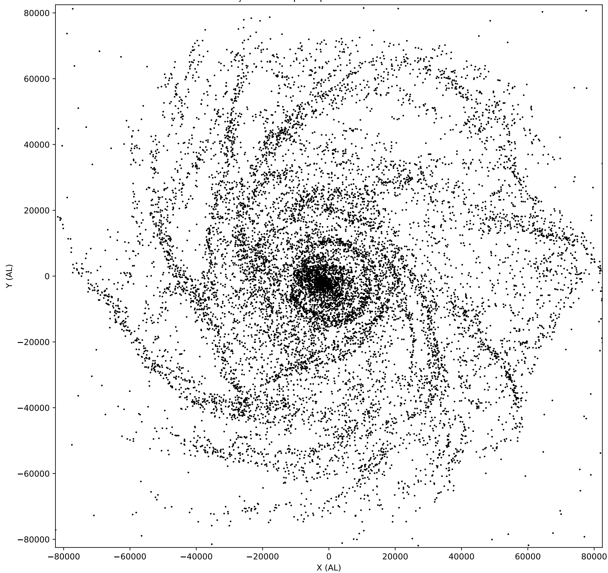
Distribuição dos corpos apos 435400.000000 milenios
