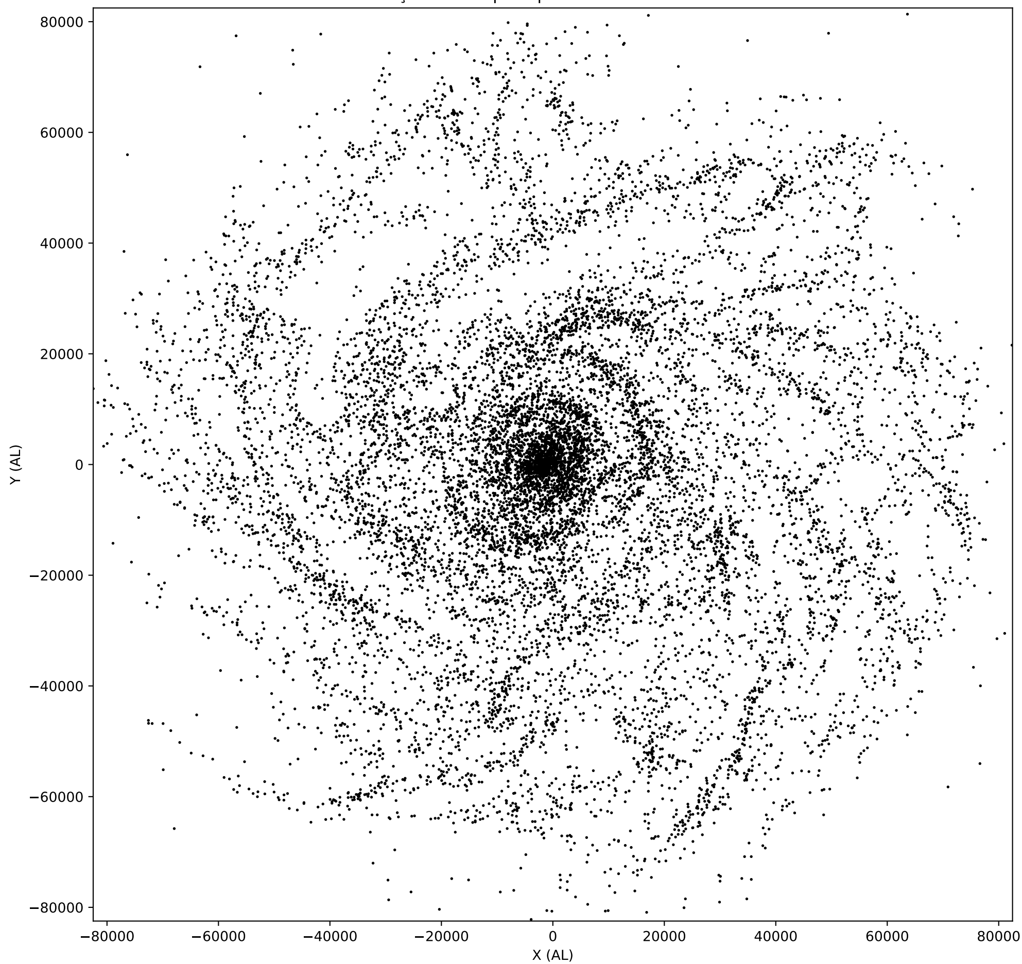
Distribuição dos corpos apos 493500.000000 milenios
