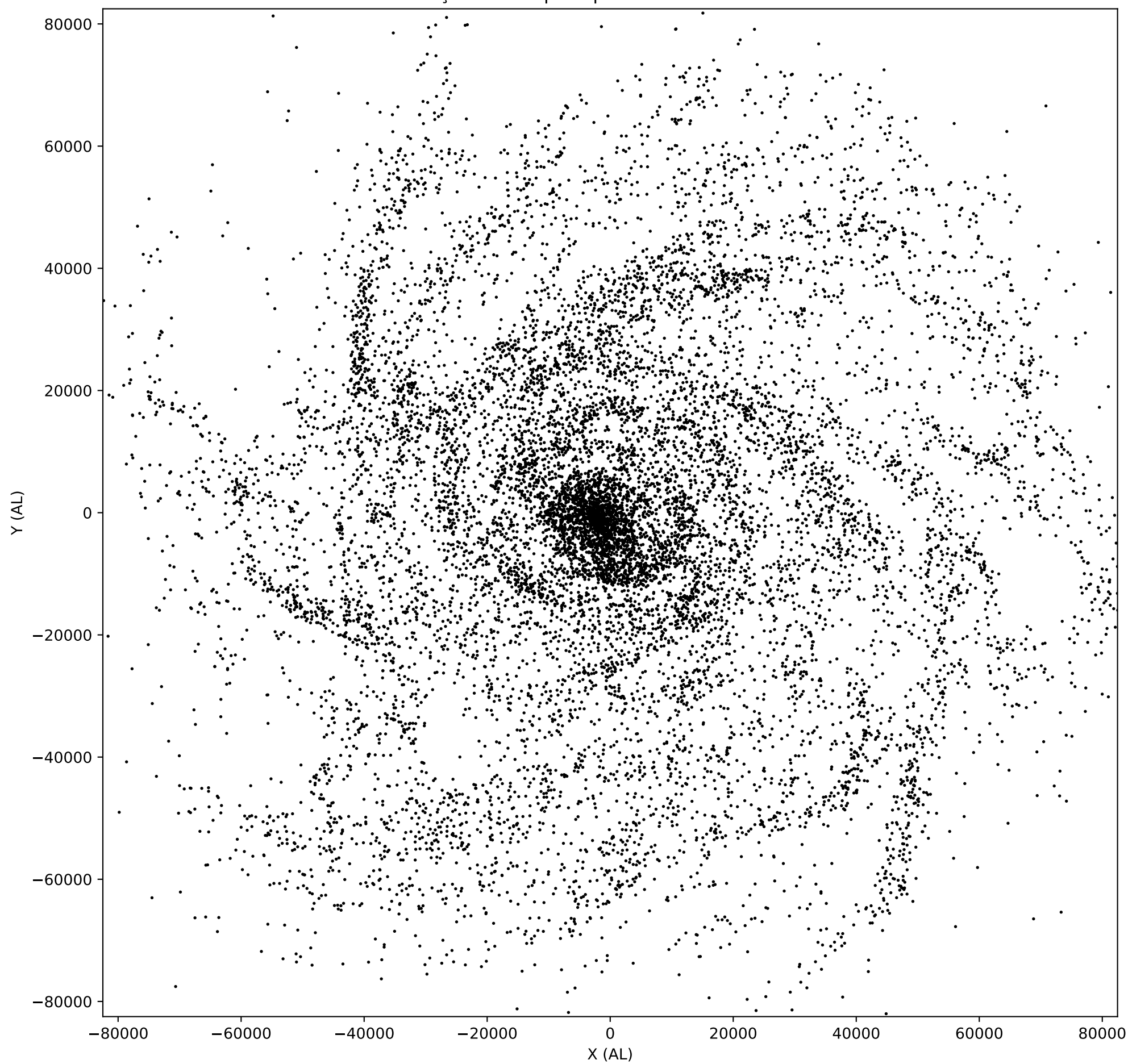
Distribuição dos corpos apos 574800.000000 milenios
