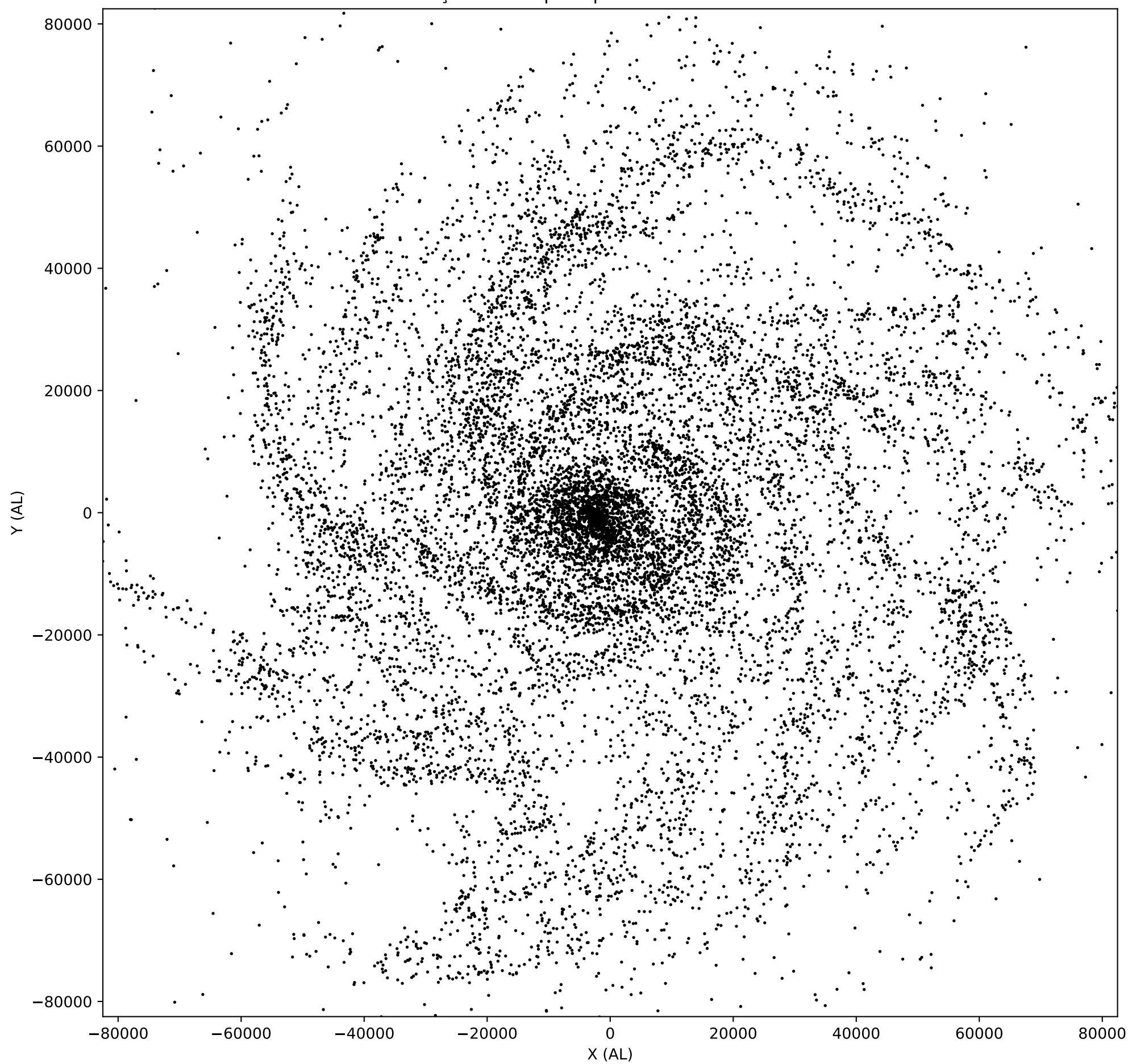
Distribuição dos corpos apos 602100.000000 milenios
