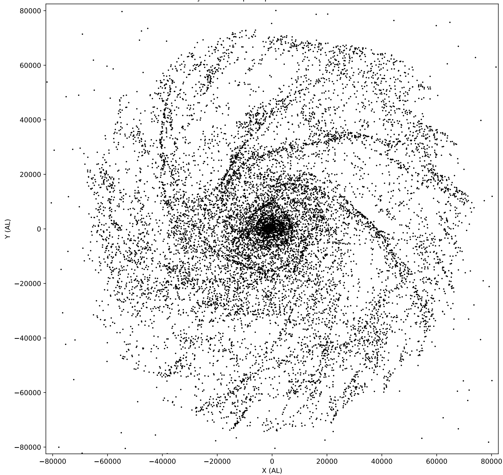
Distribuição dos corpos apos 144700.000000 milenios
