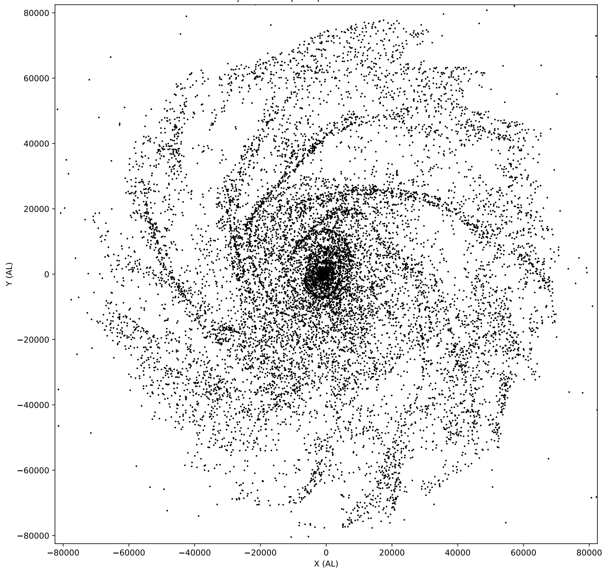
Distribuição dos corpos apos 174000.000000 milenios
