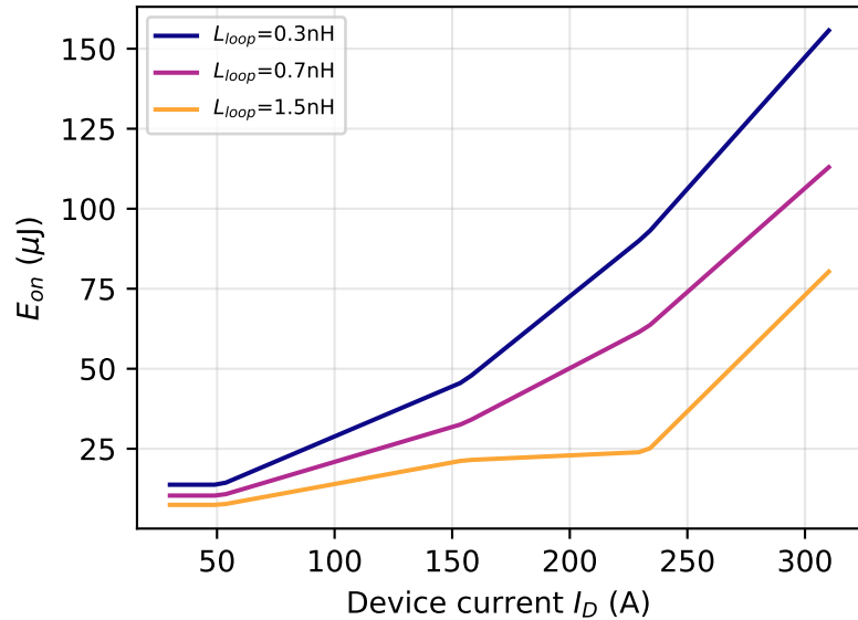
E_{on}, R_g=2\Omega
