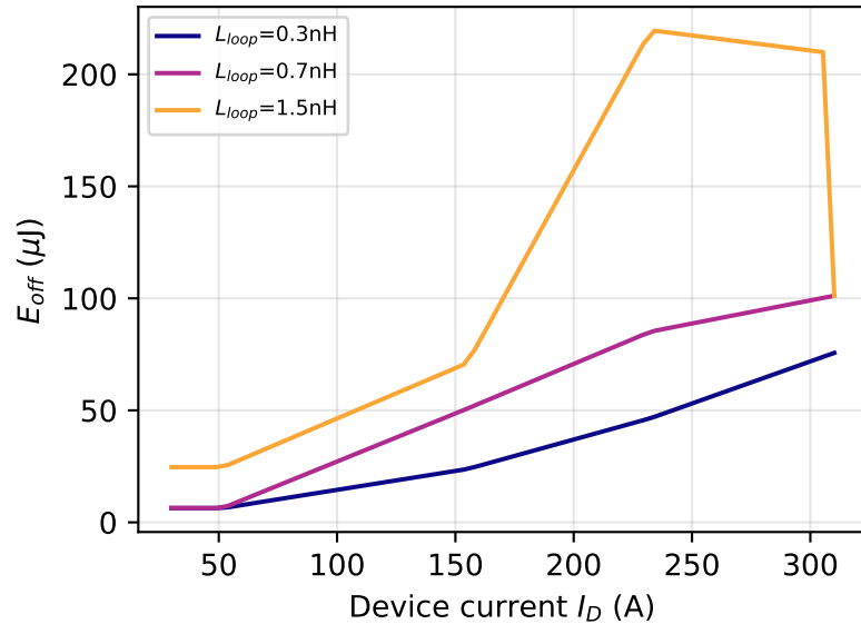
E_{off}, R_g=2\Omega
